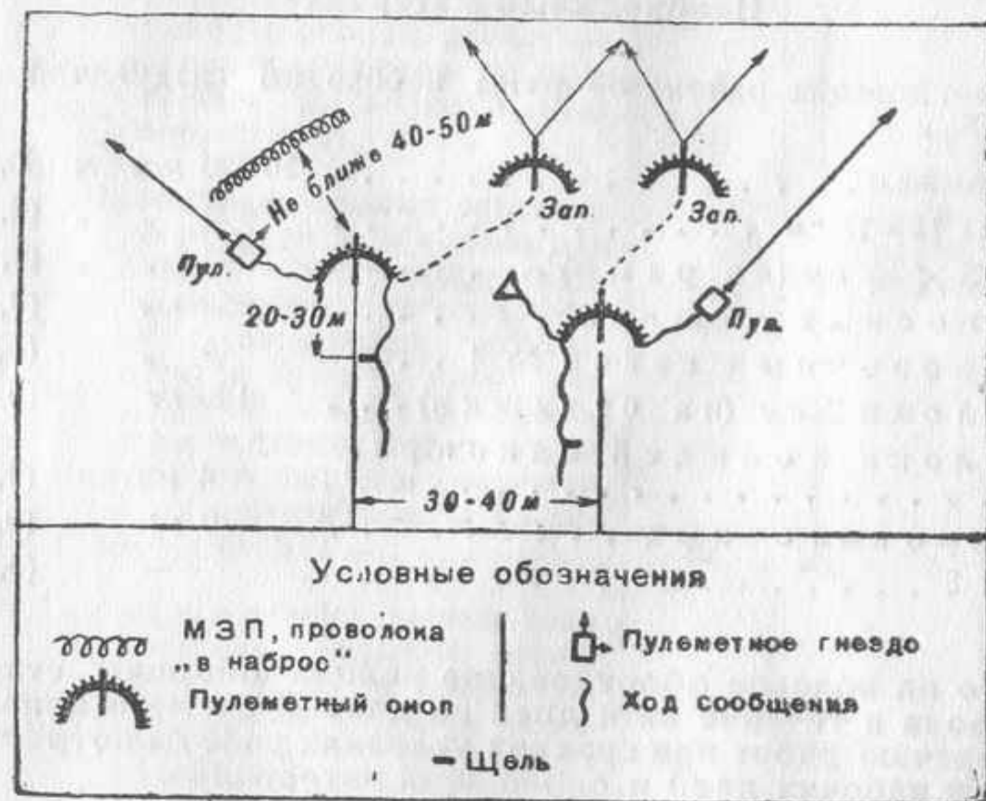
Схема позиции 1
