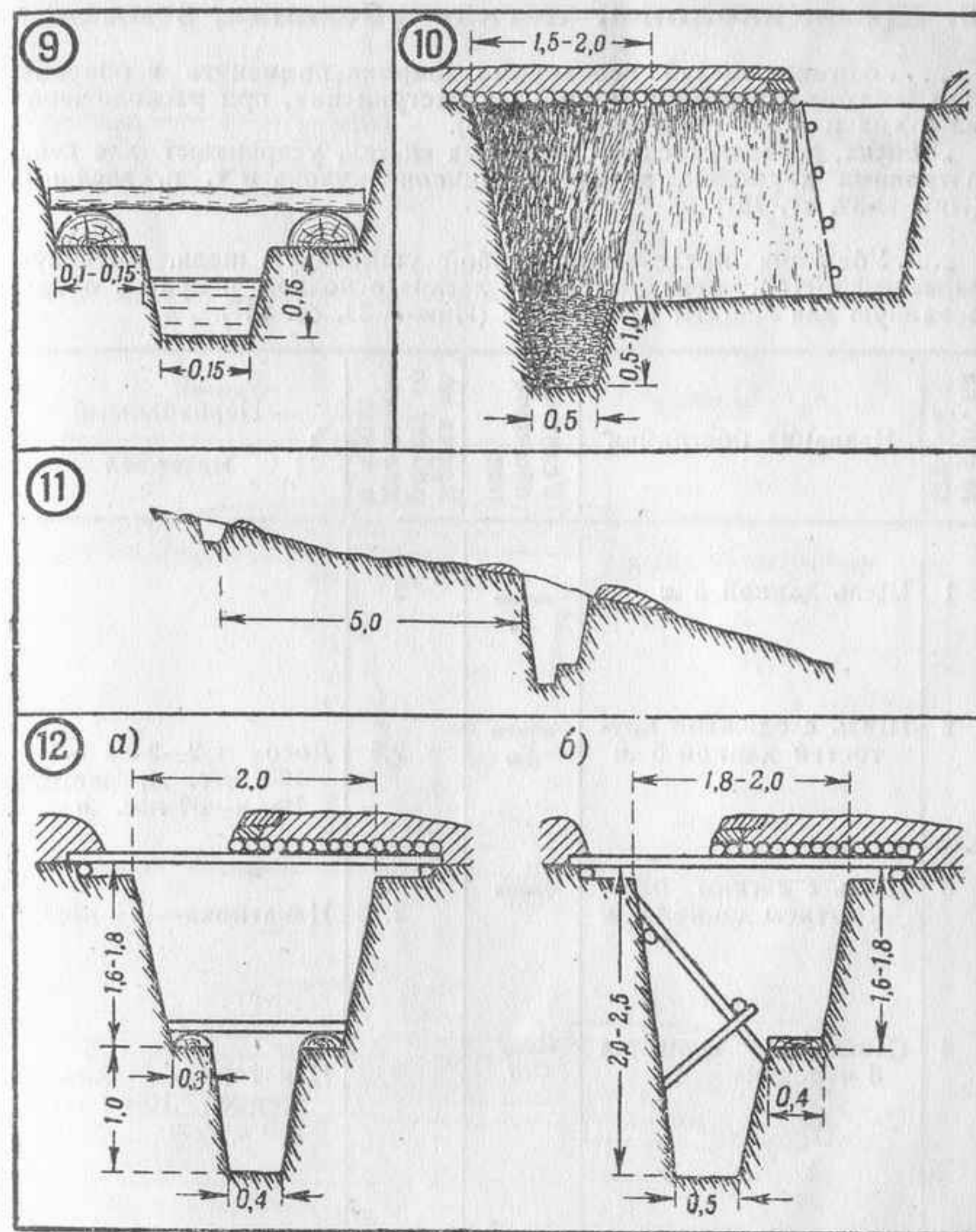
6 Укрепление местности.
