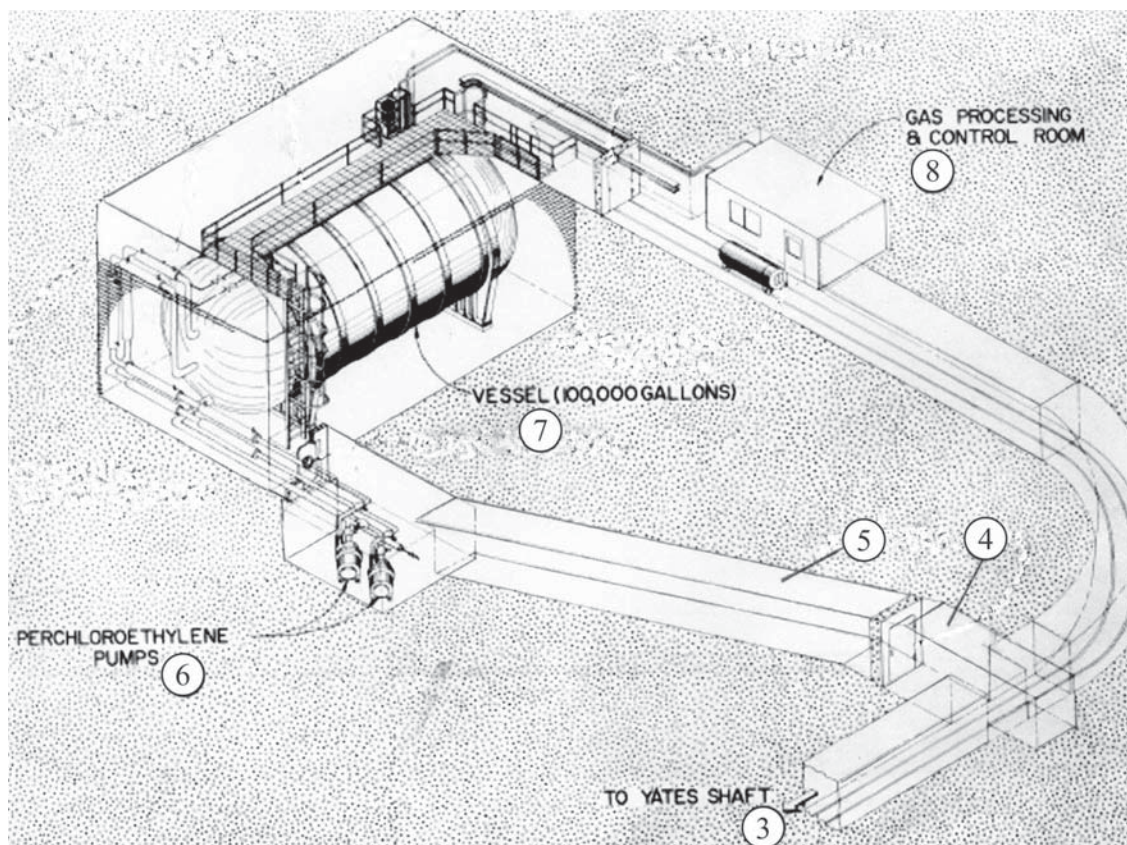
Рис. 4.24. Исследовательский комплекс нумерация позиций соответствует рис. 4.23
