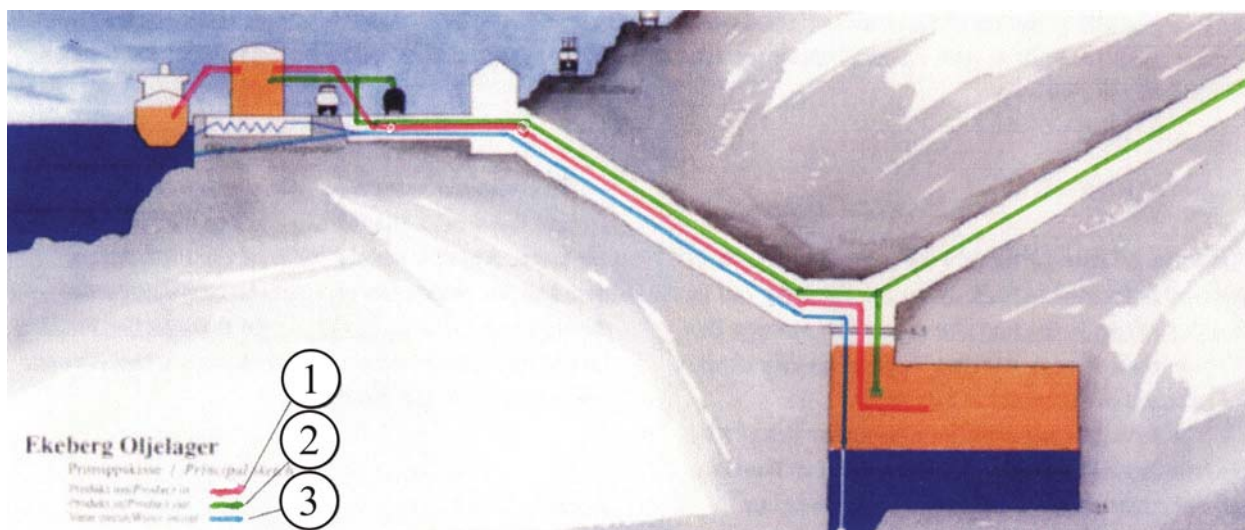
Рис. 2.15. Хранилище с постоянным уровнем топлива
