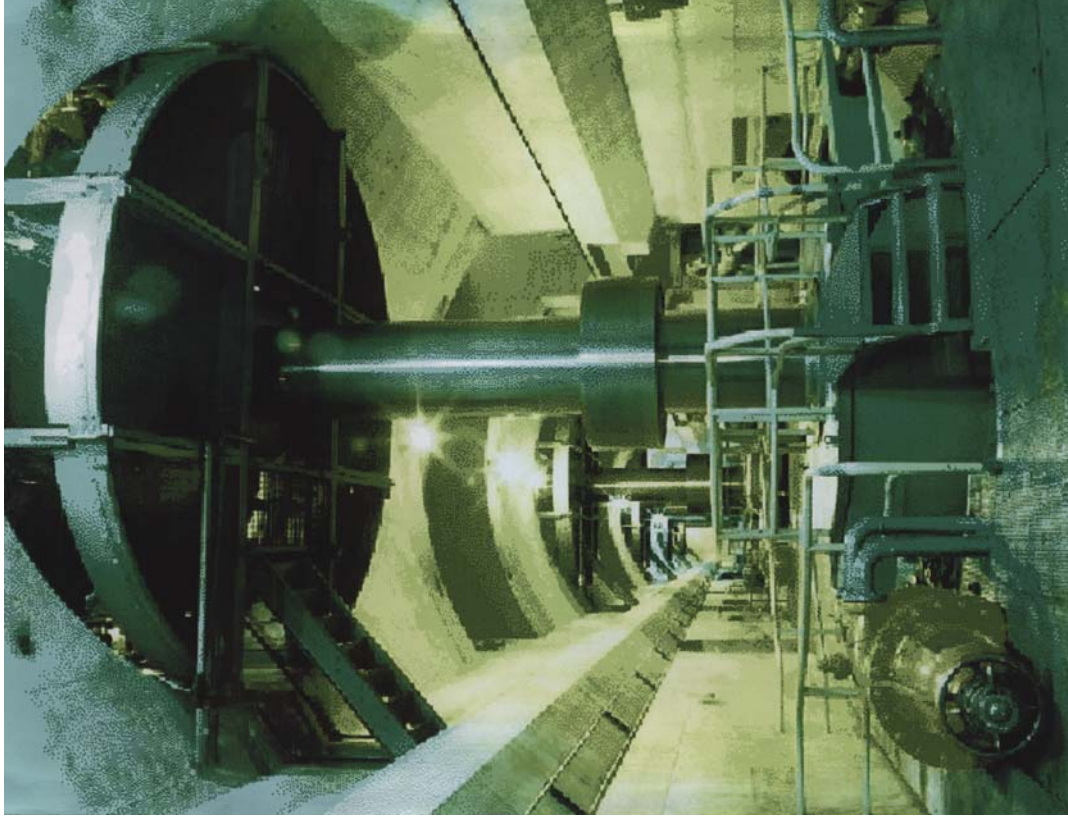
Рис. 2.37. Турбинный зал станции Динорвиг
