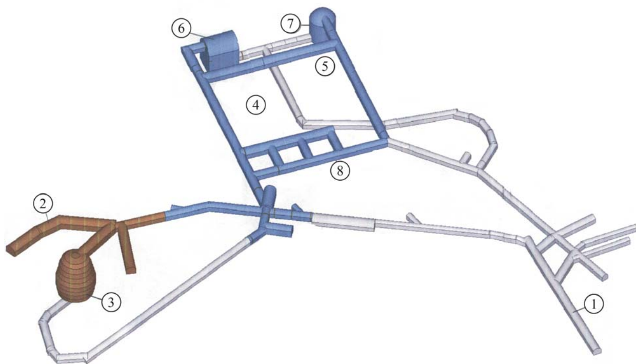
Рис. 4.72. Схема лабораторных комплексов (существующего и перспективного) шахты Крайтон
