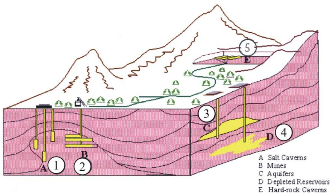
Рис. 2.1. Классификация типов хранилища природного газа
