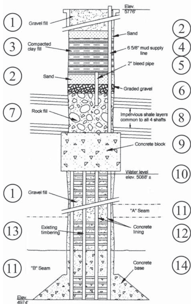
Рис. 2.20. Схема герметизации шахтного ствола
