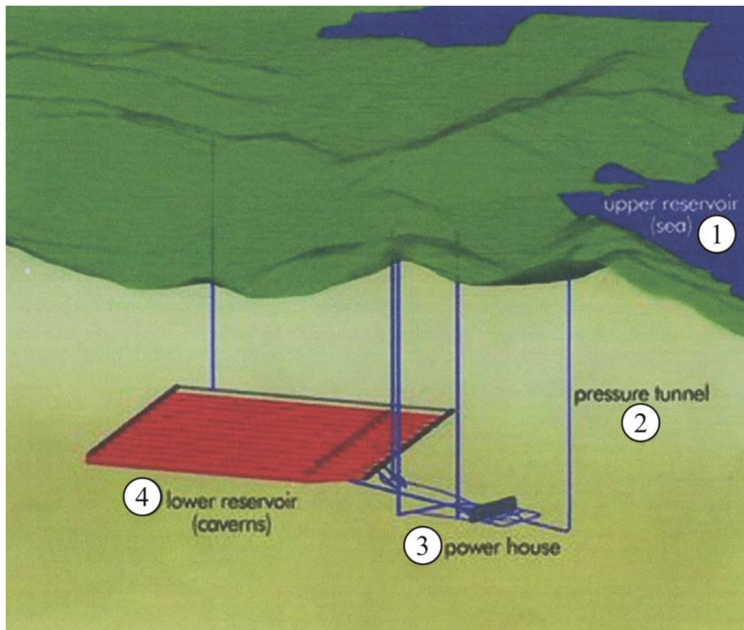
Рис. 2.40. Схема комплекса туннелей и полостей подземной гидроэлектростанции с использованием искусственно сооруженных полостей в качестве нижнего резервуара
