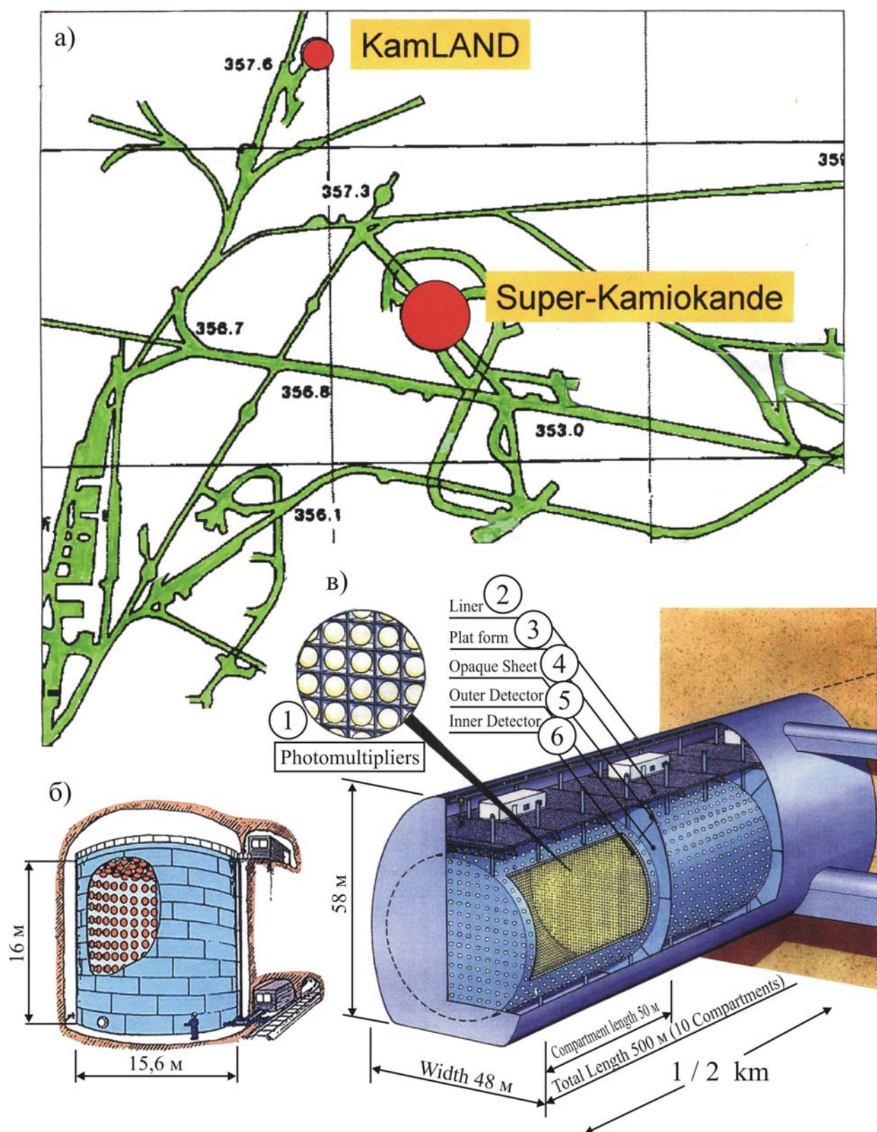
Рис. 4.40. Схема расположения научных комплексов в подземных выработках шахты Мозуми (лаборатория Камиока)
