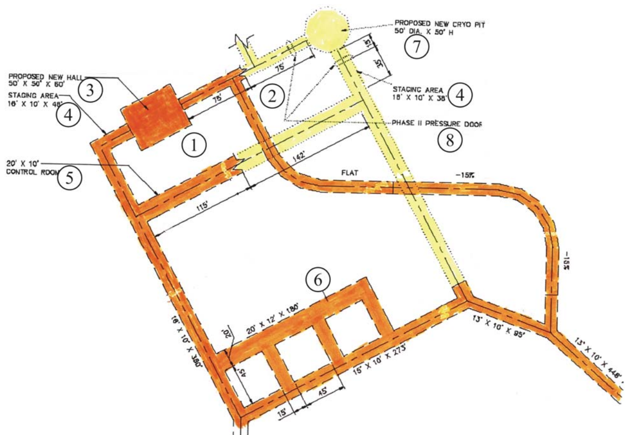
Рис. 4.71. Схема горных выработок и полостей перспективного лабораторного комплекса (размеры в футах, 1 фут = 0,3048 м) шахты Крайтон
