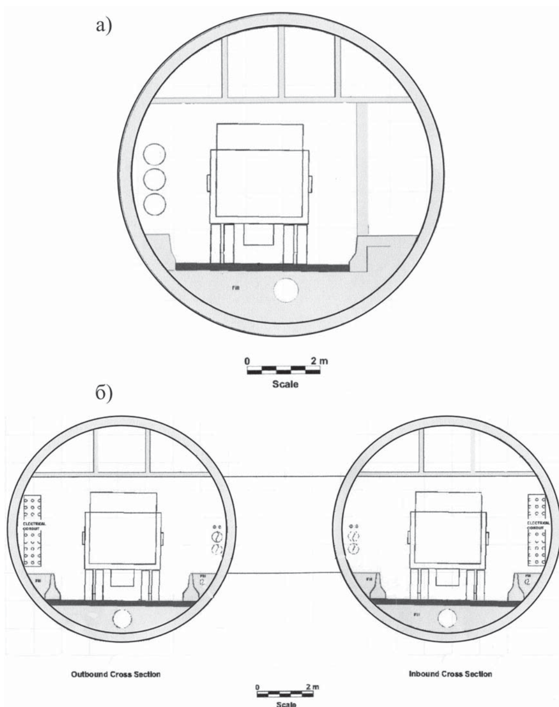
Рис. 4.35. Сечения туннелей, подводящих к научной лаборатории
