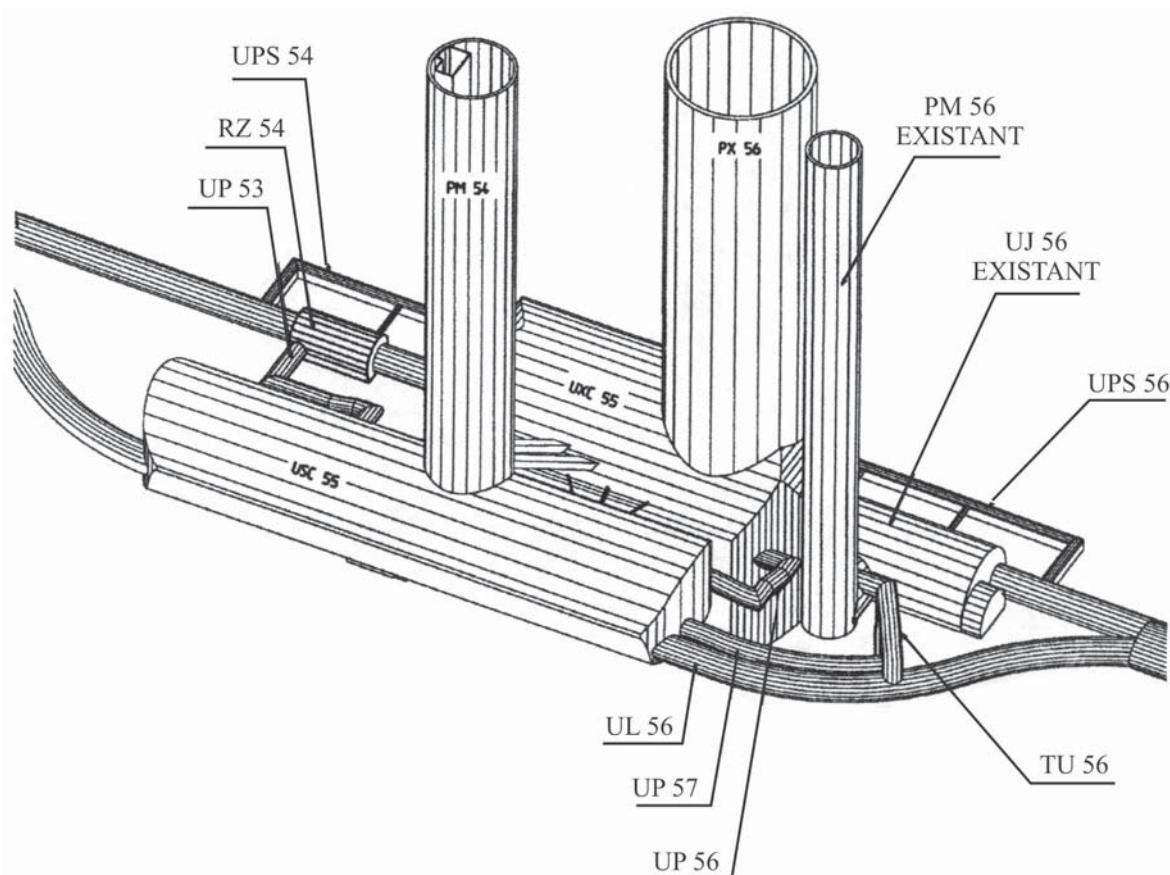
Рис. 4.96. Подземный комплекс CMS (пункт 5) реконструируемого ускорителя
