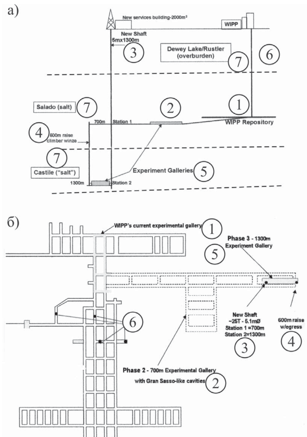
Рис. 4.29. Схемы расположения исследовательских комплексов Карлсбадской национальной лаборатории
