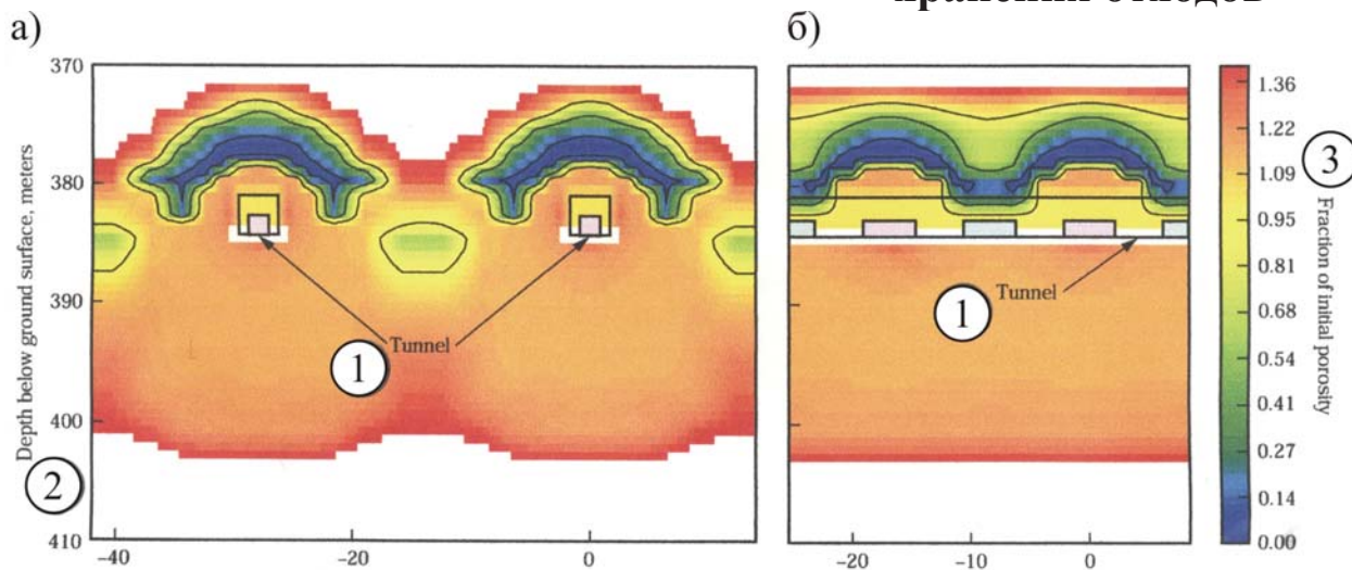
Рис. 3.50. Образование уплотненных куполов горных пород в своде туннелей хранения отходов
