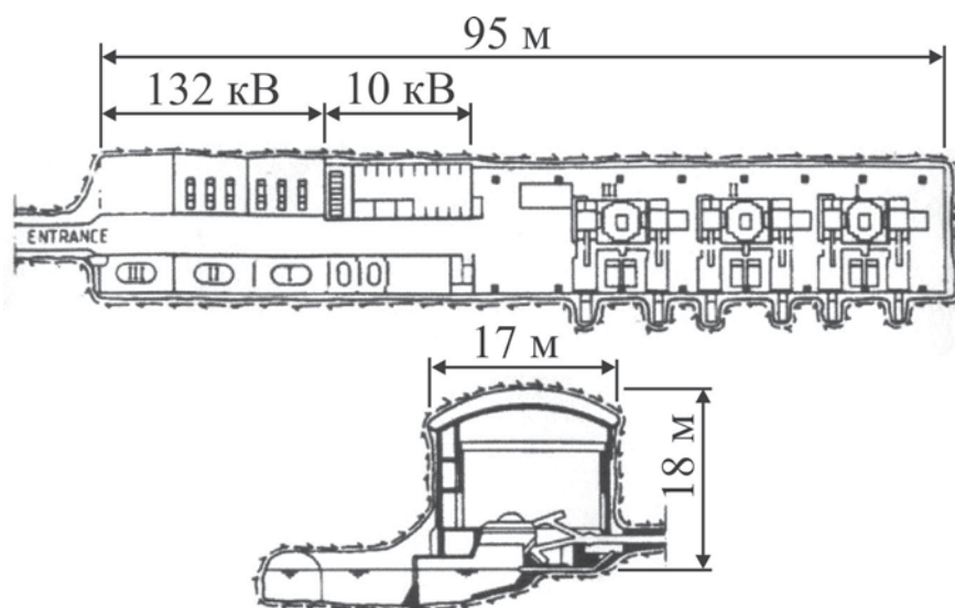
Рис. 2.47. Установка горизонтальных турбин в машинном зале электростанции Абьора
