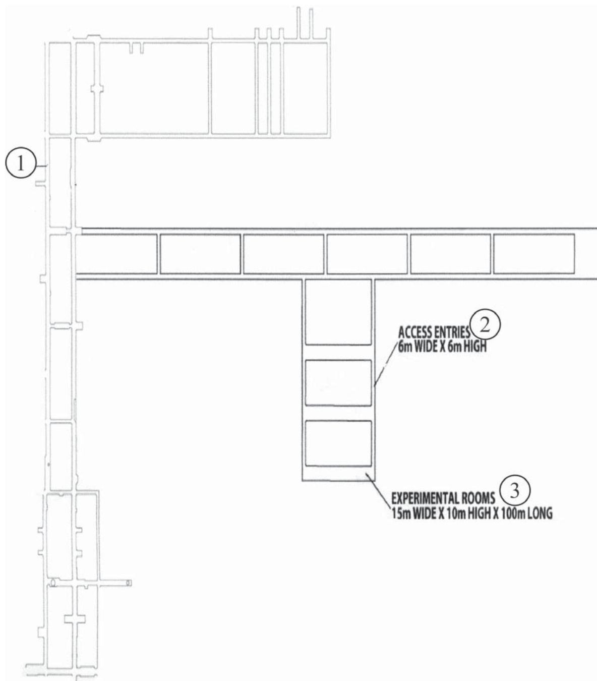
Рис. 4.30. План горных выработок на гор. 700 м – 2-я фаза комплекса лаборатории
