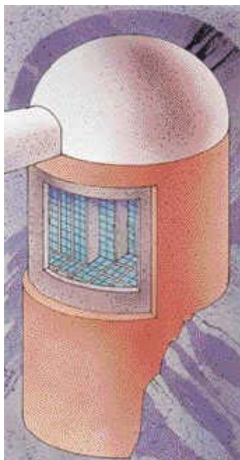
Рис. 3.31. Вертикальная скважина для хранения канистр с отходами
