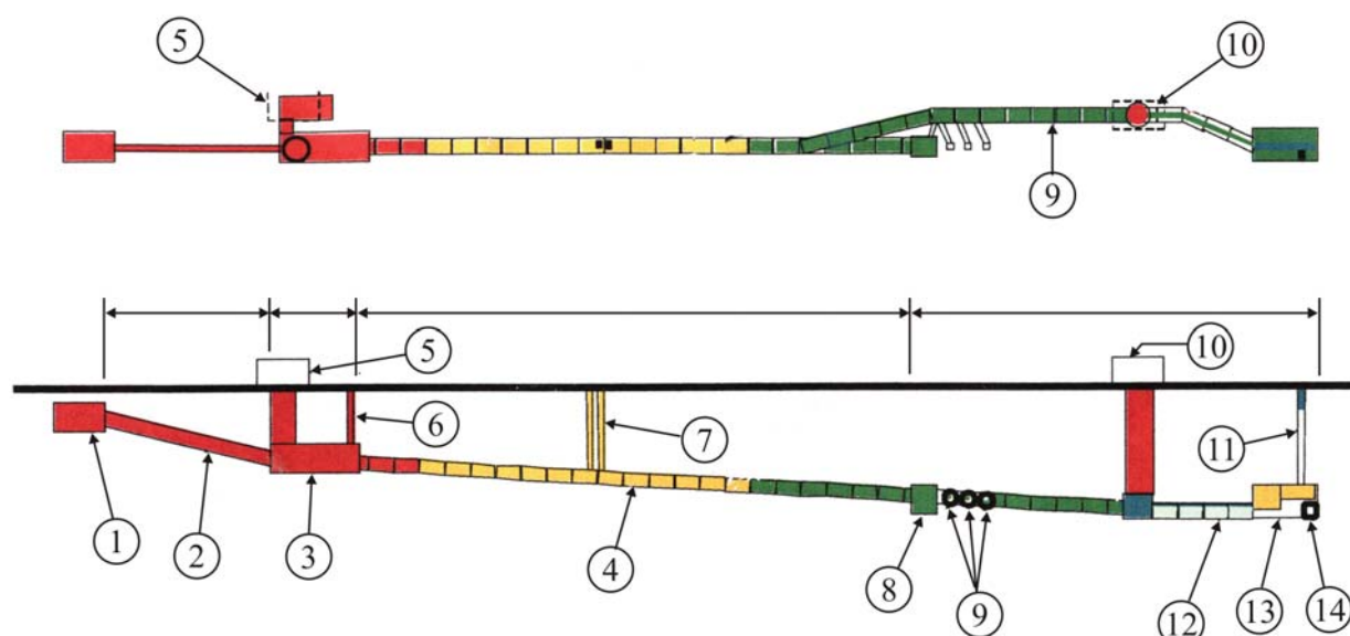
Рис. 4.8. План и разрез подземного комплекса NUMI-MINOS
