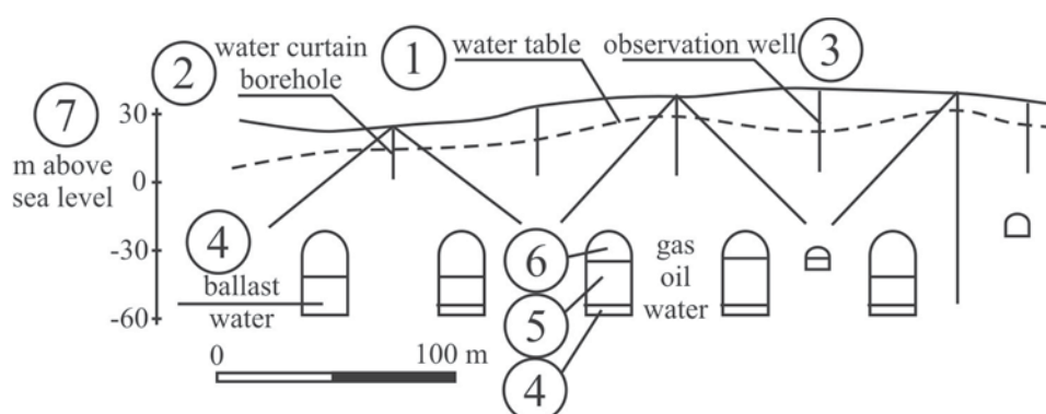
Рис. 2.14. Скважины, пробуренные для создания водной завесы 1 – уровень грунтовых вод; 2 – скважины; 3 – наблюдательные колодцы; 4 – слой балластной воды; 5 – слой нефти; 6 – слой газа; 7 – высота над уровнем моря, м
