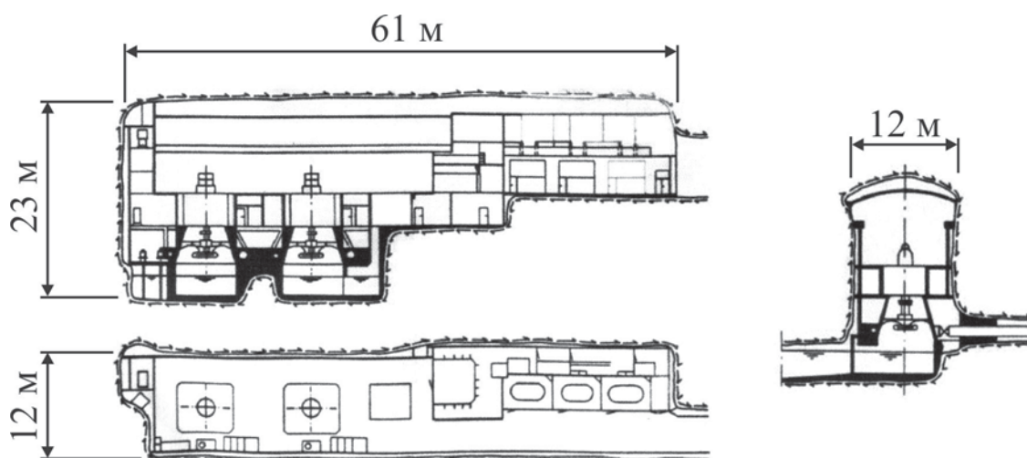
Рис. 2.48. Установка вертикальных турбин в машинном зале электростанции Хьягтдола
