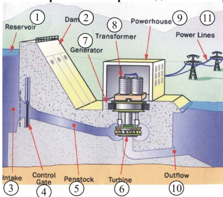
Рис. 2.30. Принципиальная схема работы генератора
