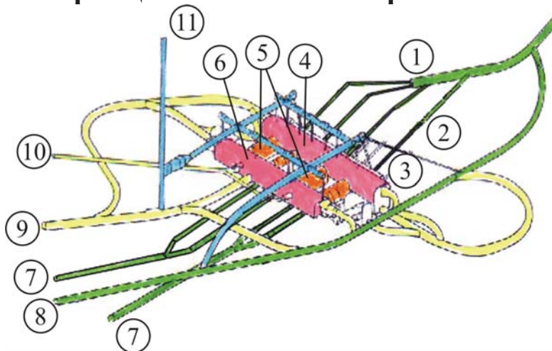
Рис. 2.31. Общая схема подземной структуры гидроаккумулирующей (насосной) электростанции (Динорвиг)
