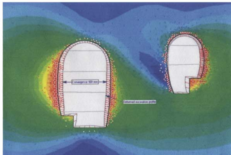
Рис. 1.7. Варианты формы сечений машинных залов гидростанции Мингтан
