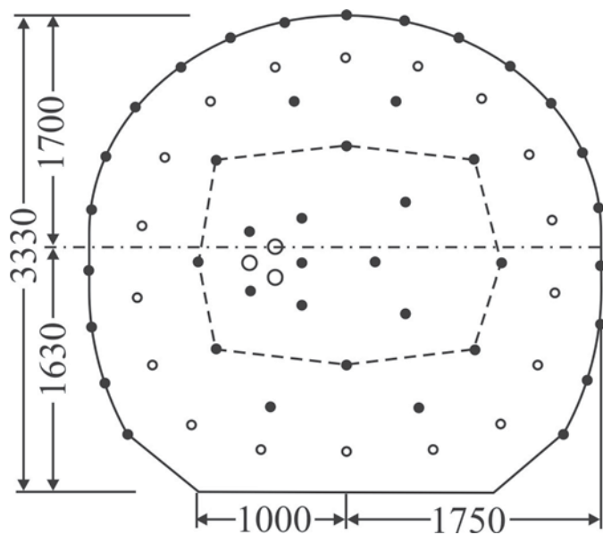
Рис. 3.45. Расположение скважин для взрывных работ в сечении туннеля
