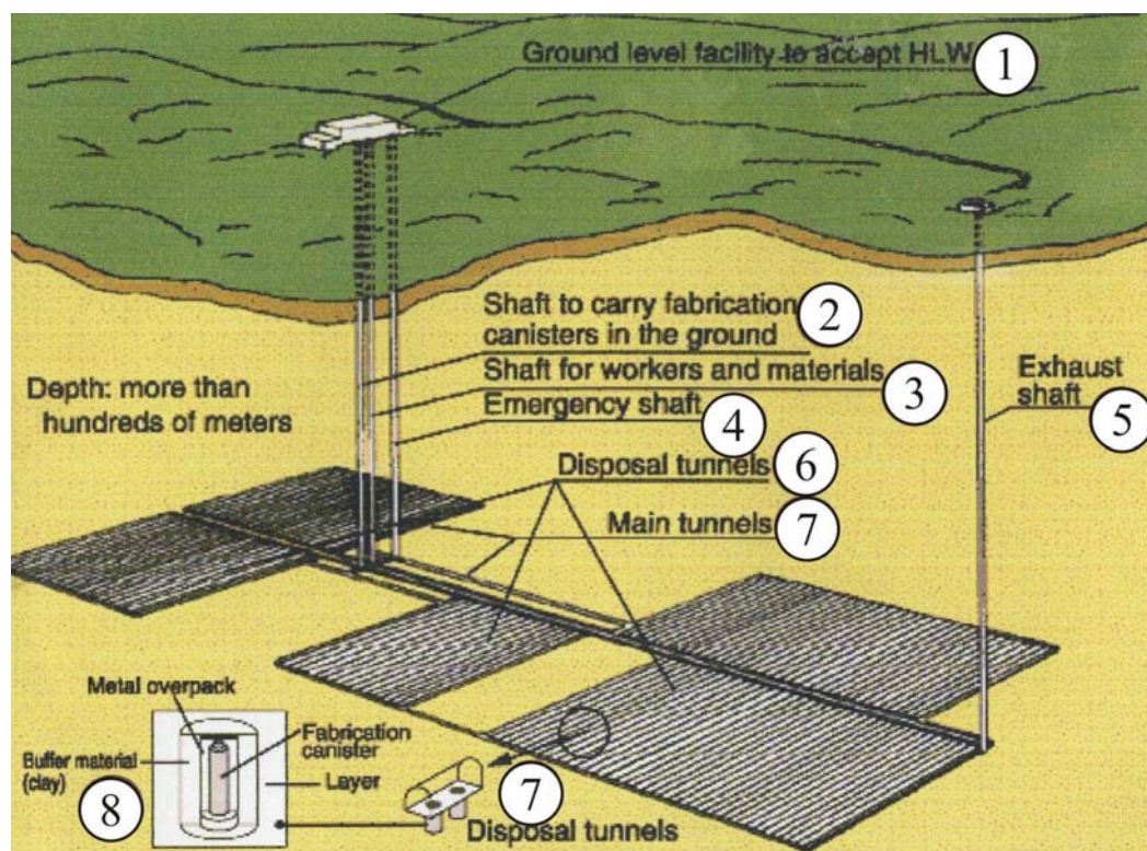
Рис. 3.39. Концепция подземного хранилища отходов с высоким уровнем радиоактивности
