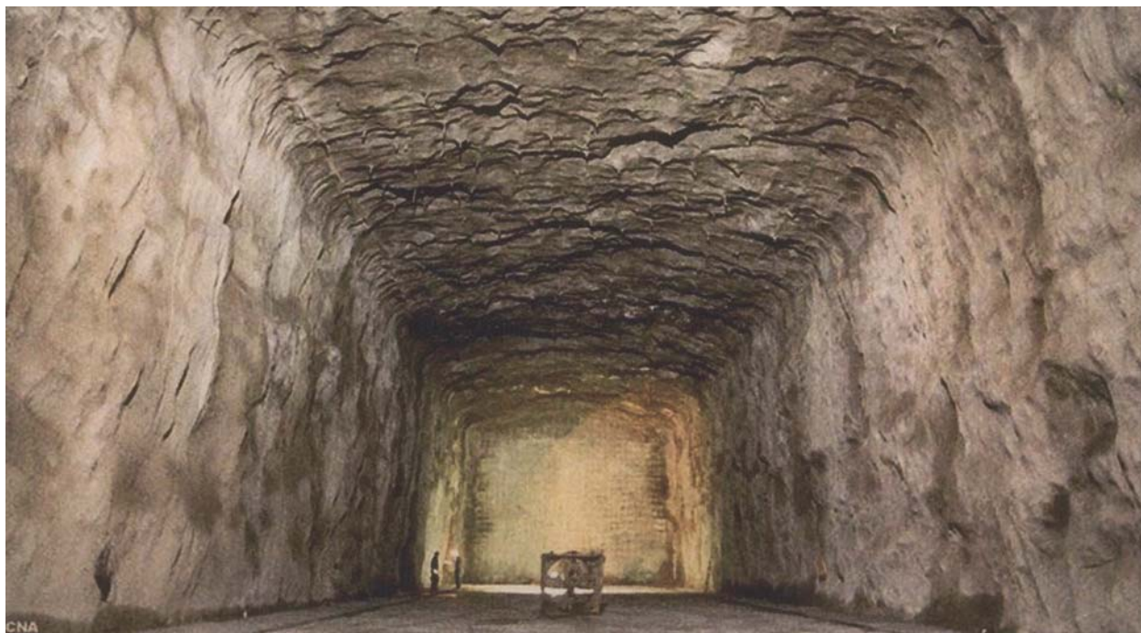
Рис. 4.13. Подземная полость лаборатории Саудан, закрепленная анкерными болтами
