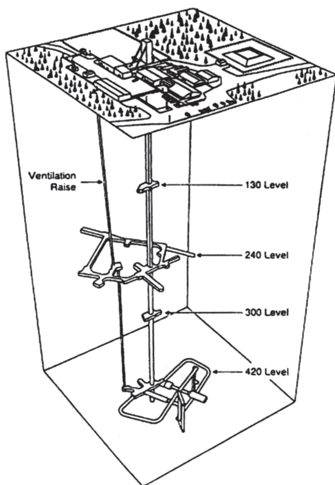
Рис. 3.44. Схема расположения основных горных выработок подземной лаборатории Манитоба
