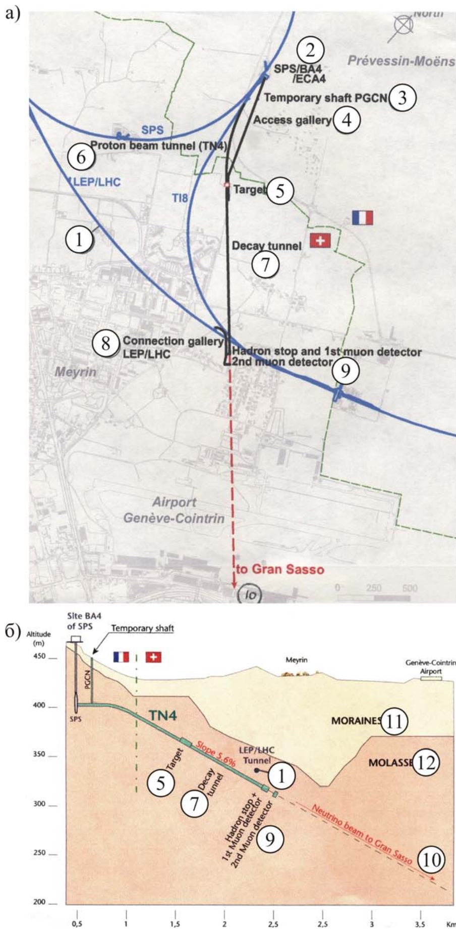
Рис. 4.111. Подземные сооружения совместного эксперимента ускорителя CERN с лабораторией Грэн Сэссо
