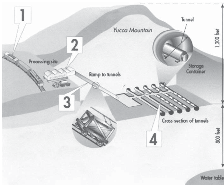
Рис. 3.18. Схемы перегрузочных операций при хранении радиоактивных отходов
