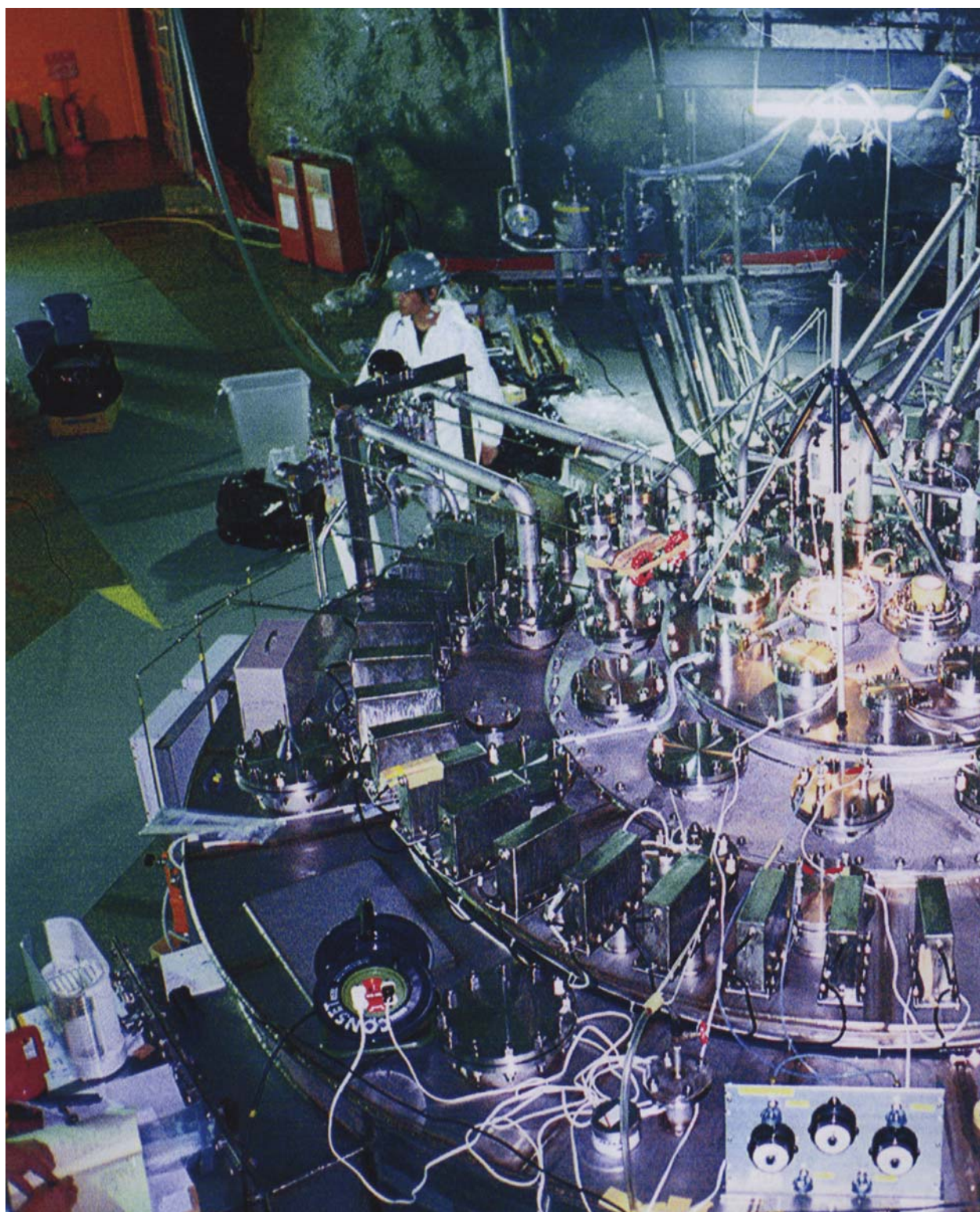
Рис. 4.42. Монтажные работы в камере детектора KamLAND
