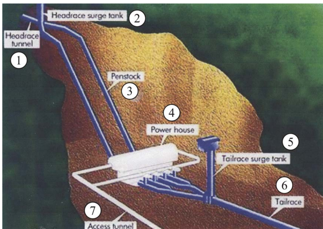
Рис. 2.45. Изометрическая схема комплекса туннелей и полостей подземной гидроэлектростанции
