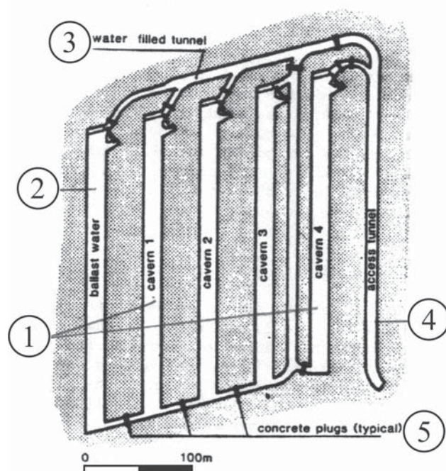
Рис. 2.13. Хранилище нефти в Стуре
