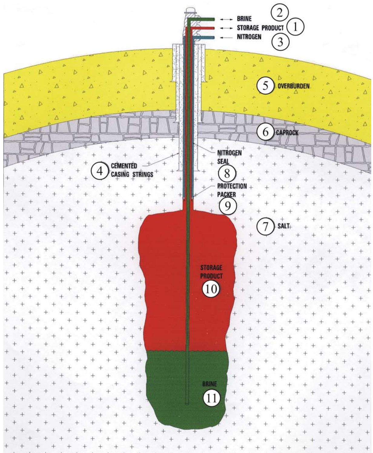
Рис. 2.5. Хранение продуктов в соляной полости
