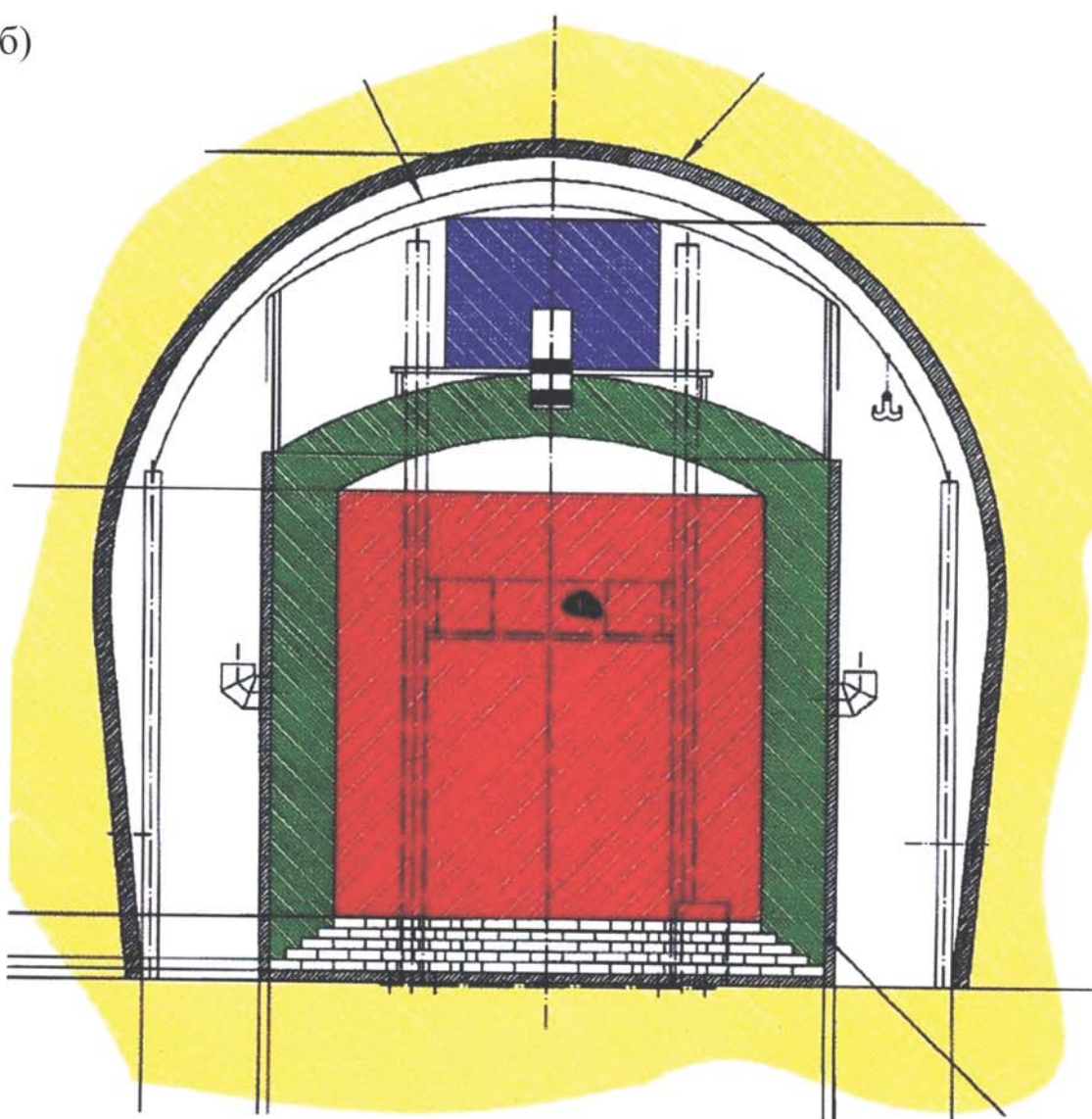
Рис. 4.81. Схемы расположения оборудования в лабораторных залах
