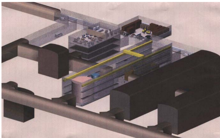
Рис. 4.37. Макет одного из вариантов подземных помещений лаборатории Сан-Джасинто
