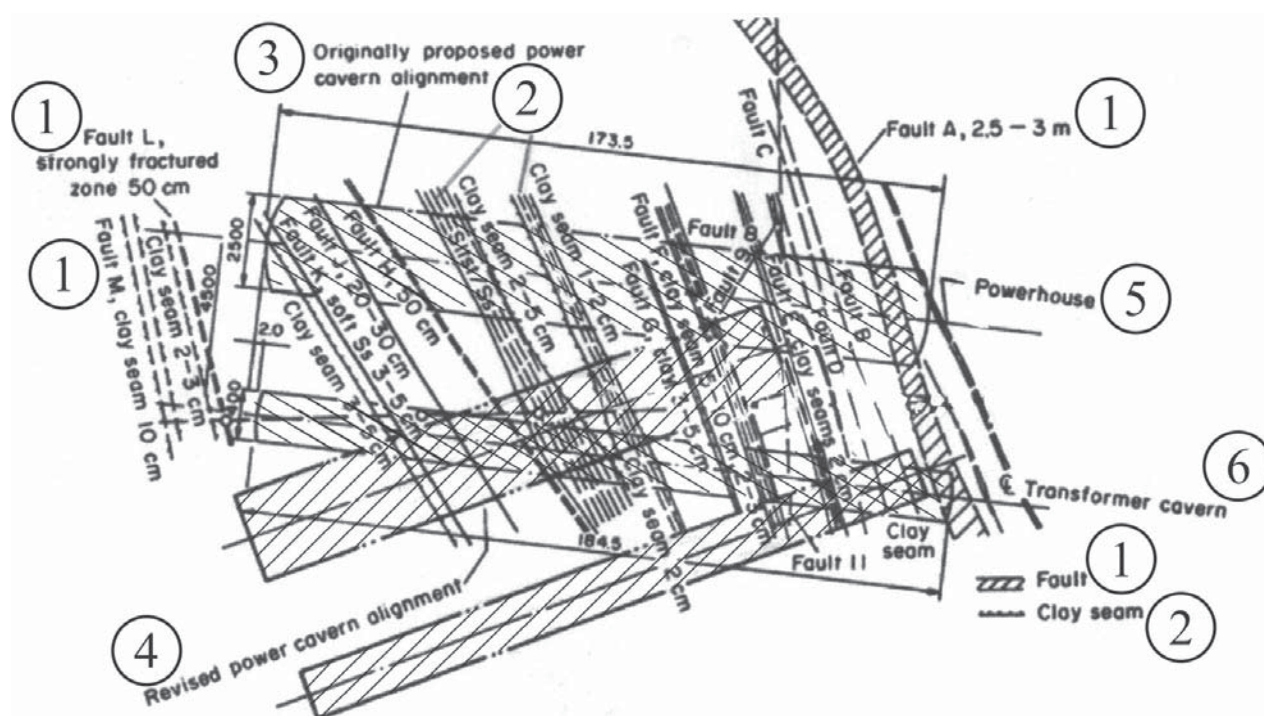
Рис. 1.5. Разворот подземного комплекса гидростанции Мингтан перпендикулярно плоскости зон нарушений
