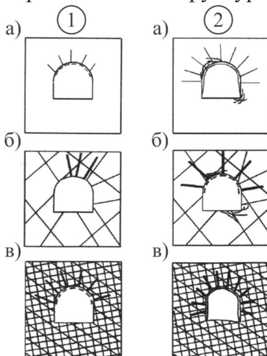
Рис. 1.20. Варианты установки анкерной крепи
