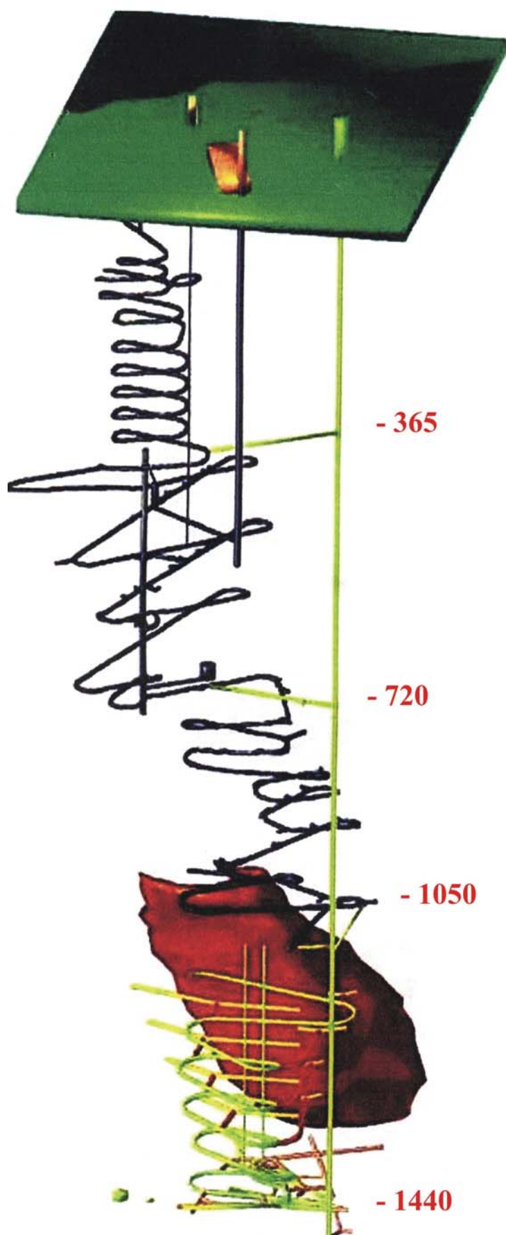
Рис. 4.50. Комплекс вскрывающих выработок существующей и новой (углубляемой) частей шахты Пихасалми
