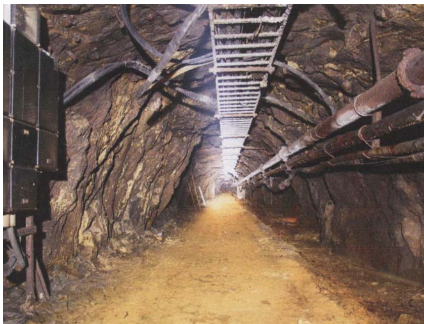
Рис. 4.49. Полость на гор. 210 м шахты Пихасалми
