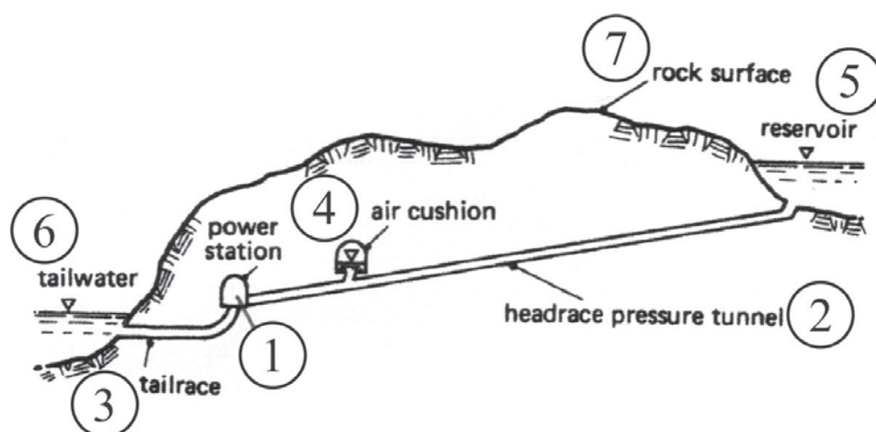
Рис. 2.52. Привязка амортизирующей камеры к комплексу туннелей и полостей гидроэлектростанции
