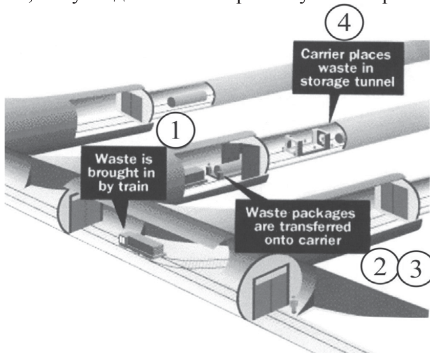
Рис. 3.19. Схемы перегрузочных операций при хранении радиоактивных отходов
