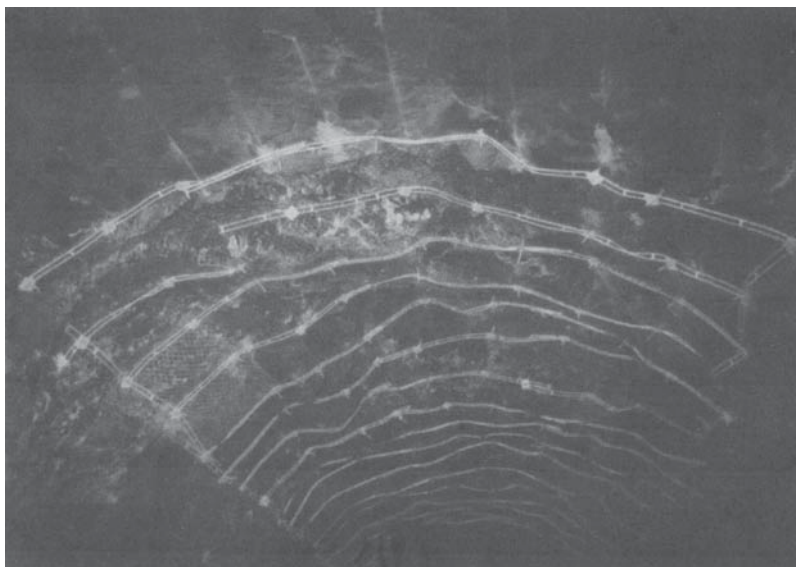
Рис. 1.16. Стальные полосы на анкерных болтах, поддерживающие кровлю полости
