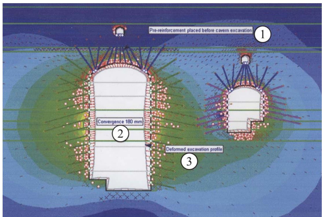
Рис. 1.9. Цифровая модель, показывающая потерю несущей способности породного массива и деформацию контуров полости
