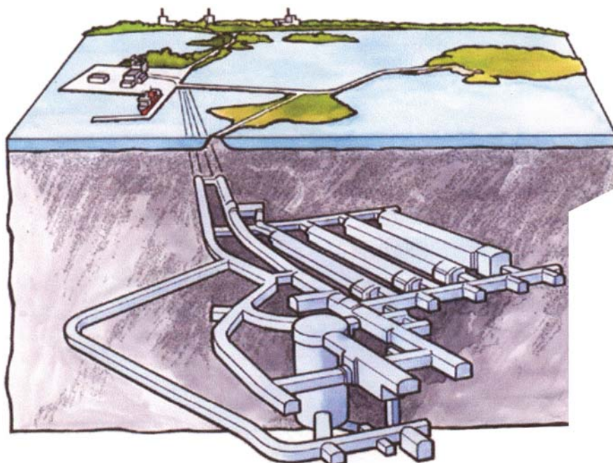
Рис. 3.28. Комплекс подземного хранения SFR (Швеция)
