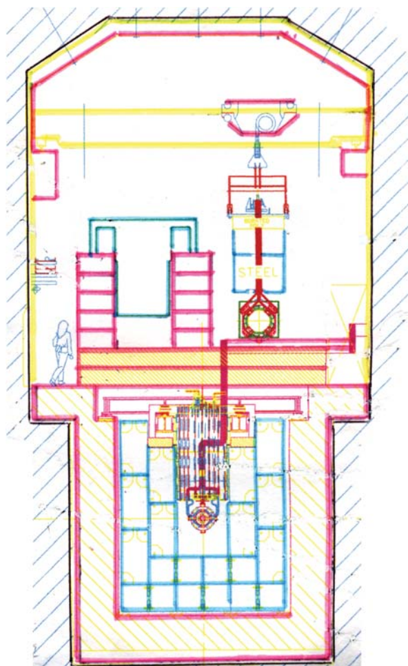
Рис. 4.17. Размещение оборудования в зале мишени («Target Hall») лаборатории Фермилаб
