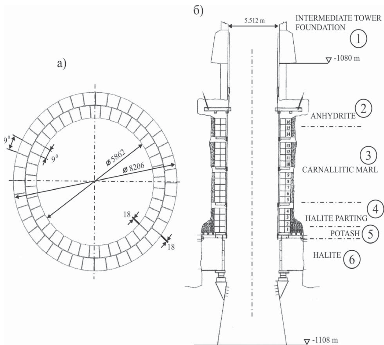
Рис. 4.65. Вторая реконструкция крепи клетового ствола
