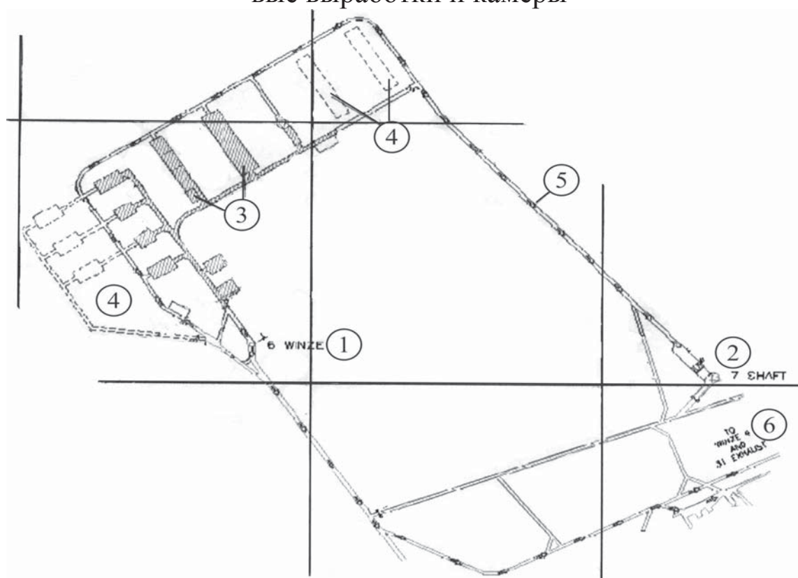
Рис. 4.27. Вариант размещения лабораторного комплекса на горизонте 7400 ф
