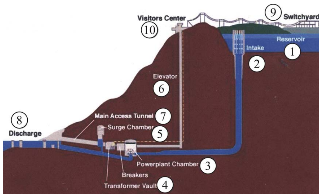
Рис. 2.46. Разрез по комплексу подземной гидроэлектростанции
