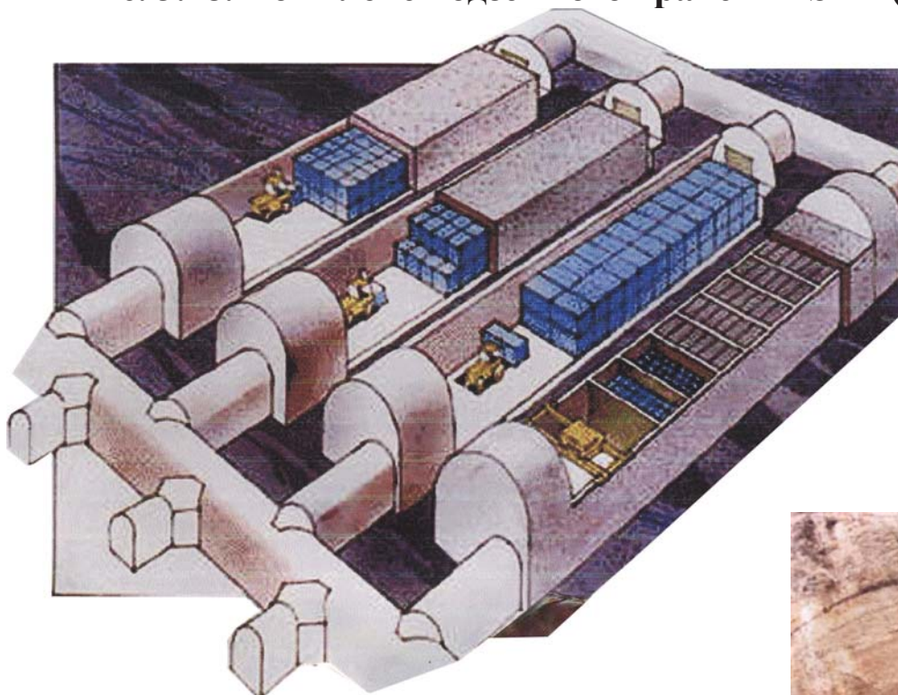
Рис. 3.29. Горизонтальные хранилища комплекса SFR
