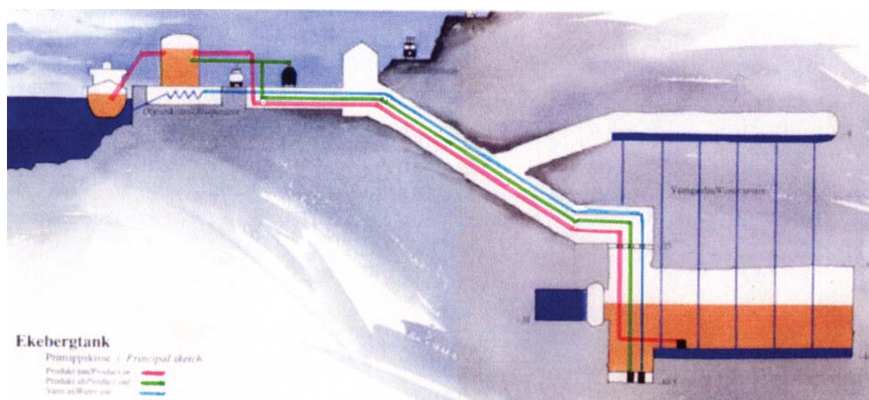
Рис. 2.16. Хранилище с переменным уровнем топлива
