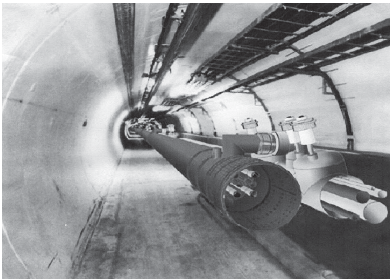
Рис. 4.94. Расположение оборудования в туннеле ускорителя
