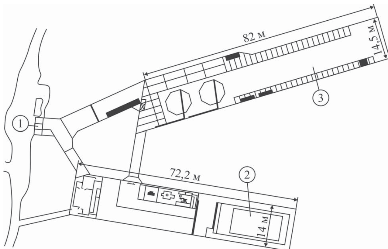
Рис. 4.2. Подземный лабораторный комплекс Саудан-2
