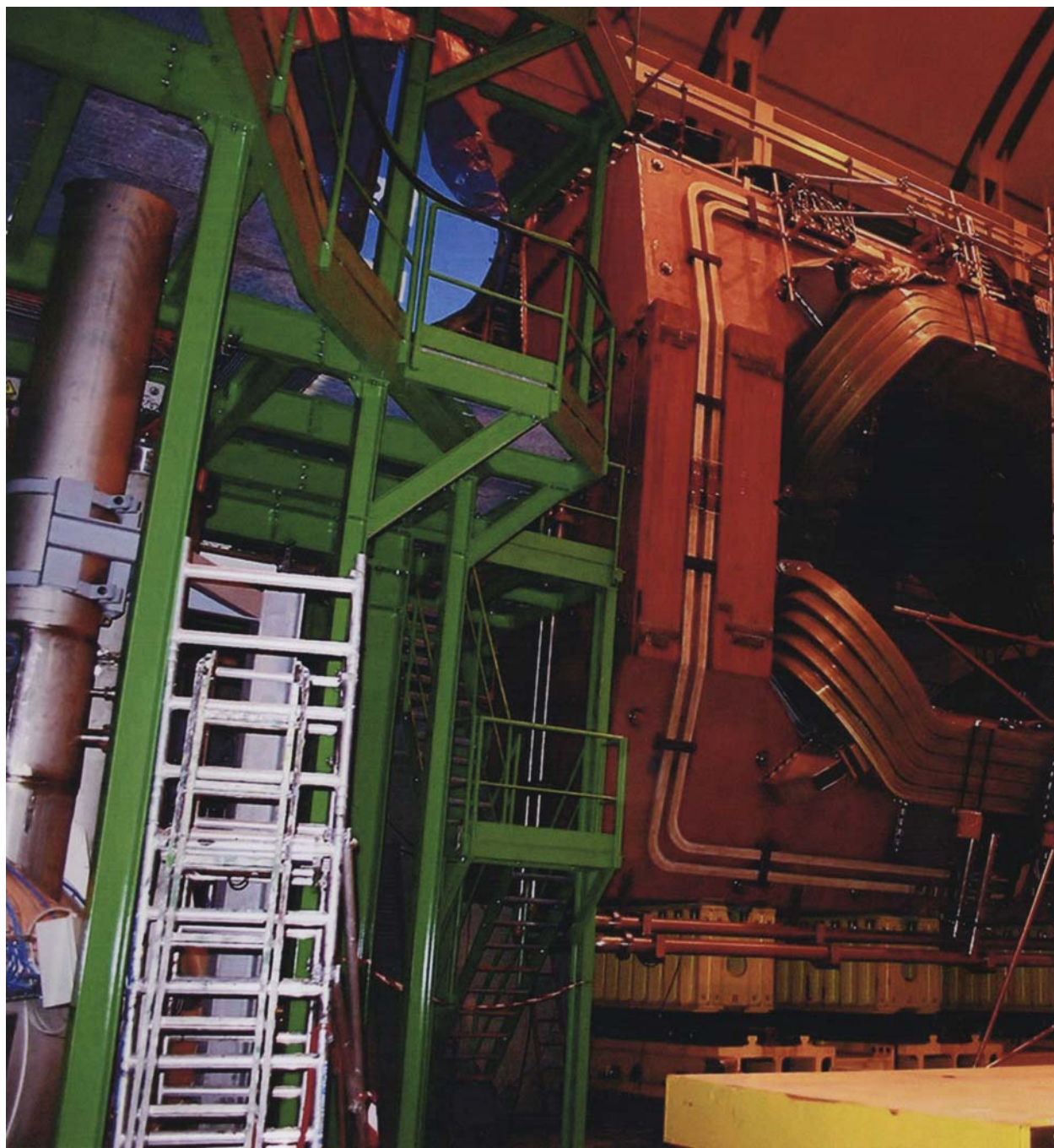
Рис. 4.109. Камера одного из магнитов ускорителя LEP/LHC
