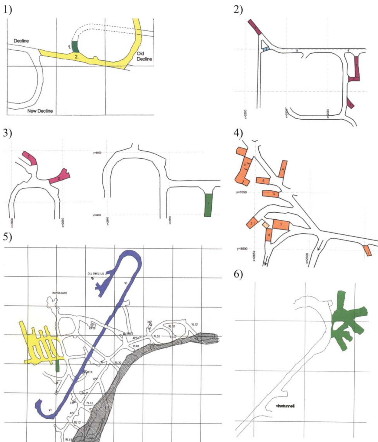
Рис. 4.53. Расположение научных комплексов различного назначения на действующих горизонтах шахты Пихасалми
