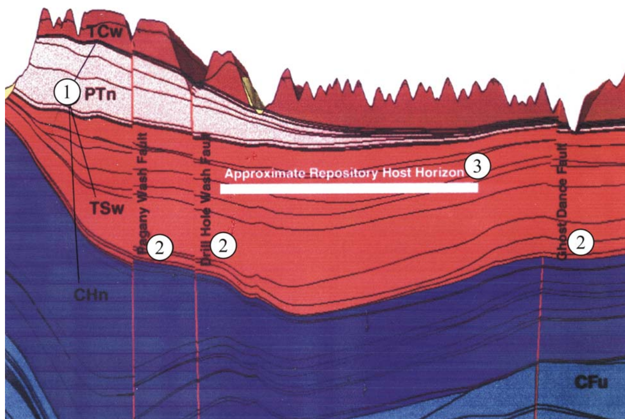
Рис. 3.8. Геологический разрез в районе строительства хранилища Юкка Маунтейн
