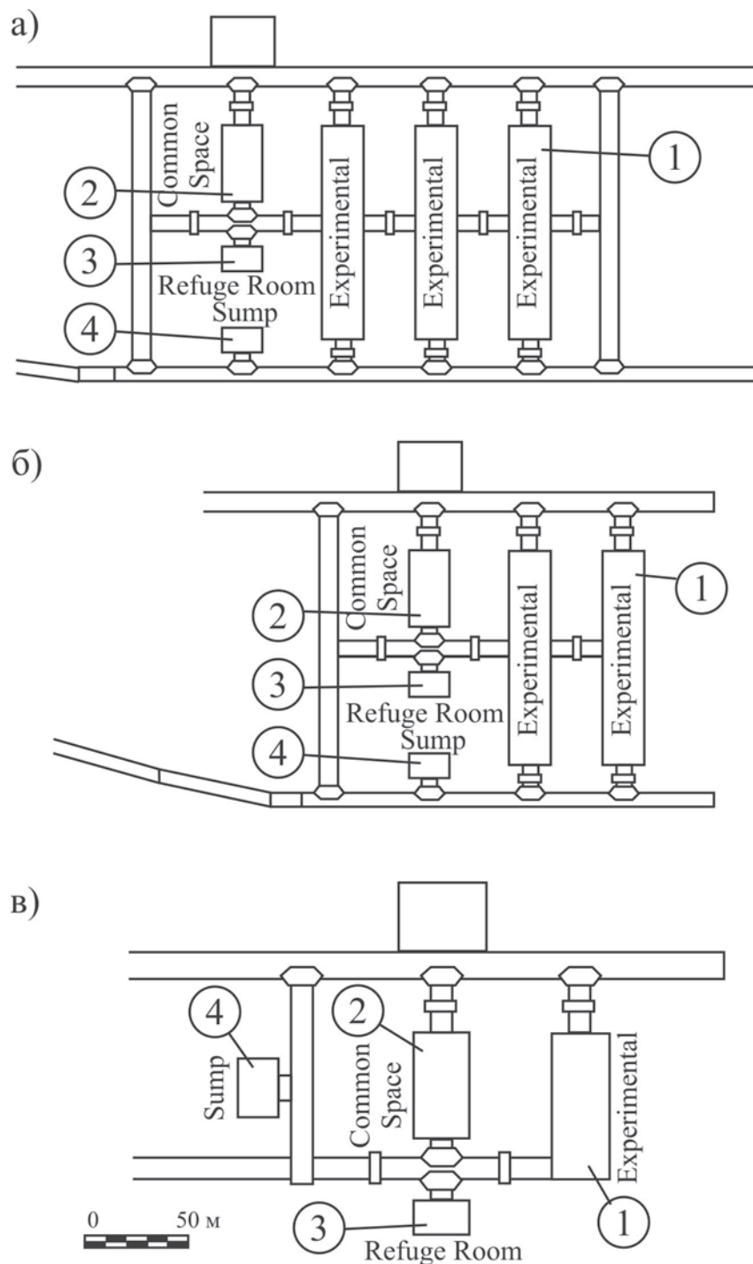
Рис. 4.36. Варианты лабораторного комплекса
