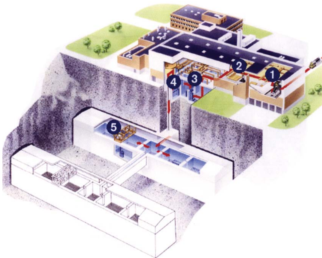
Рис. 3.32. Комплекс подземного хранилища СЛАВ (Швеция)
