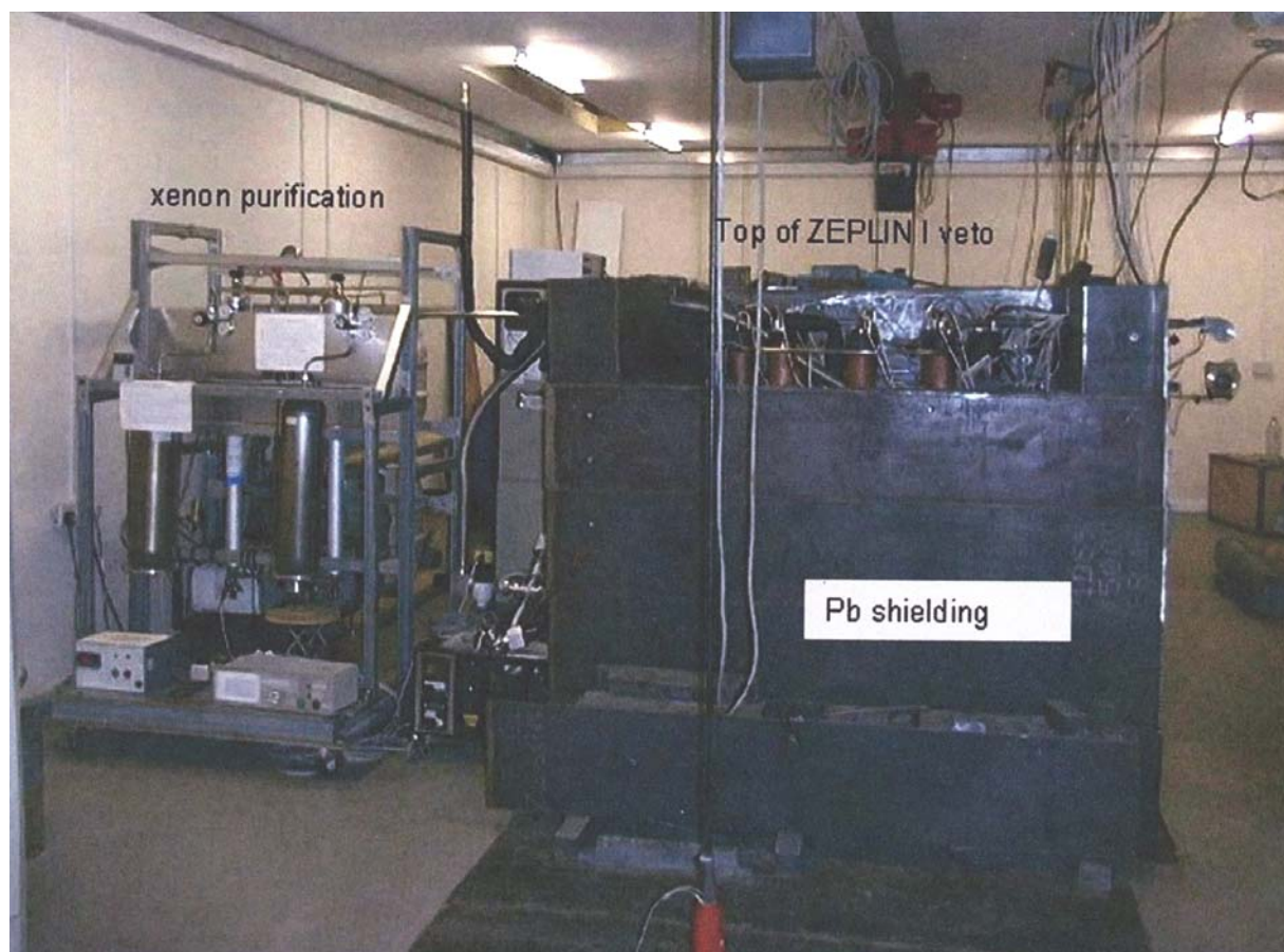
Рис. 4.58. Установка детектора Zeplin в подземной лаборатории
