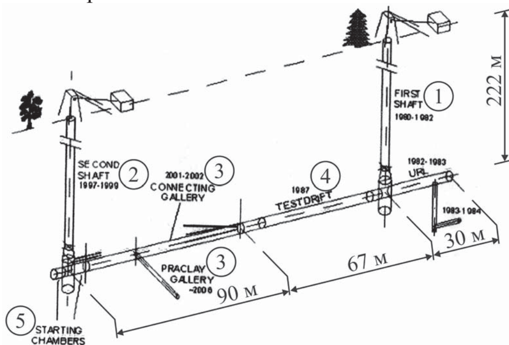
Рис. 3.47. Схема основных горных выработок подземной лаборатории Хейдес
