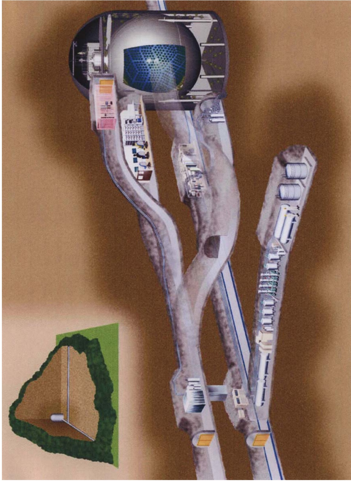
Рис. 4.41. Схема установки детектора KamLAND в шахте Мозуми
