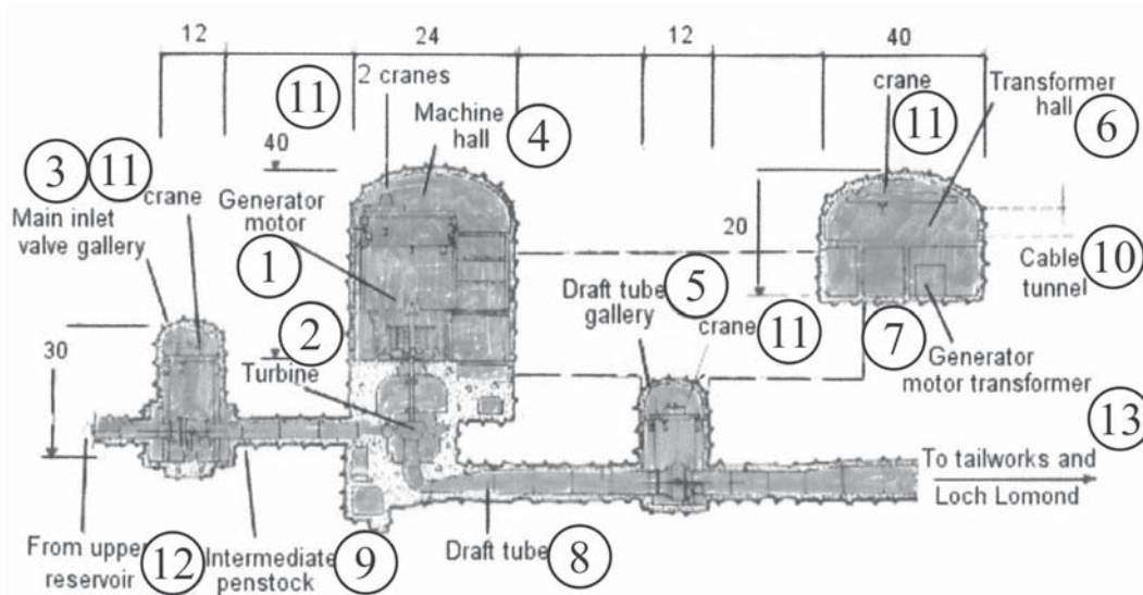
Рис. 2.32. Комплекс главных подземных полостей гидроаккумулирующей электростанции (Динорвиг)
