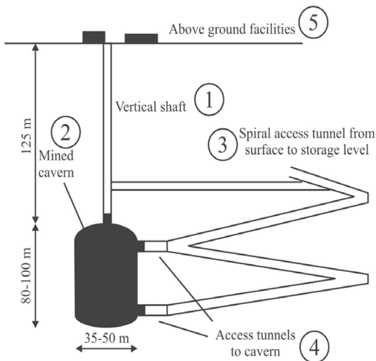
Рис. 2.7. Закрепленная полость, пройденная шахтным способом 1 – вертикальная шахта; 2 – закрепленная полость; 3 – спиральный туннель доступа с поверхности к горизонту хранения; 4 – туннели доступа к полости; 5 – наземные здания и сооружения
