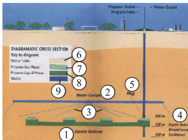
Рис. 2.8. Общая схема подземного хранилища сжиженного газа
