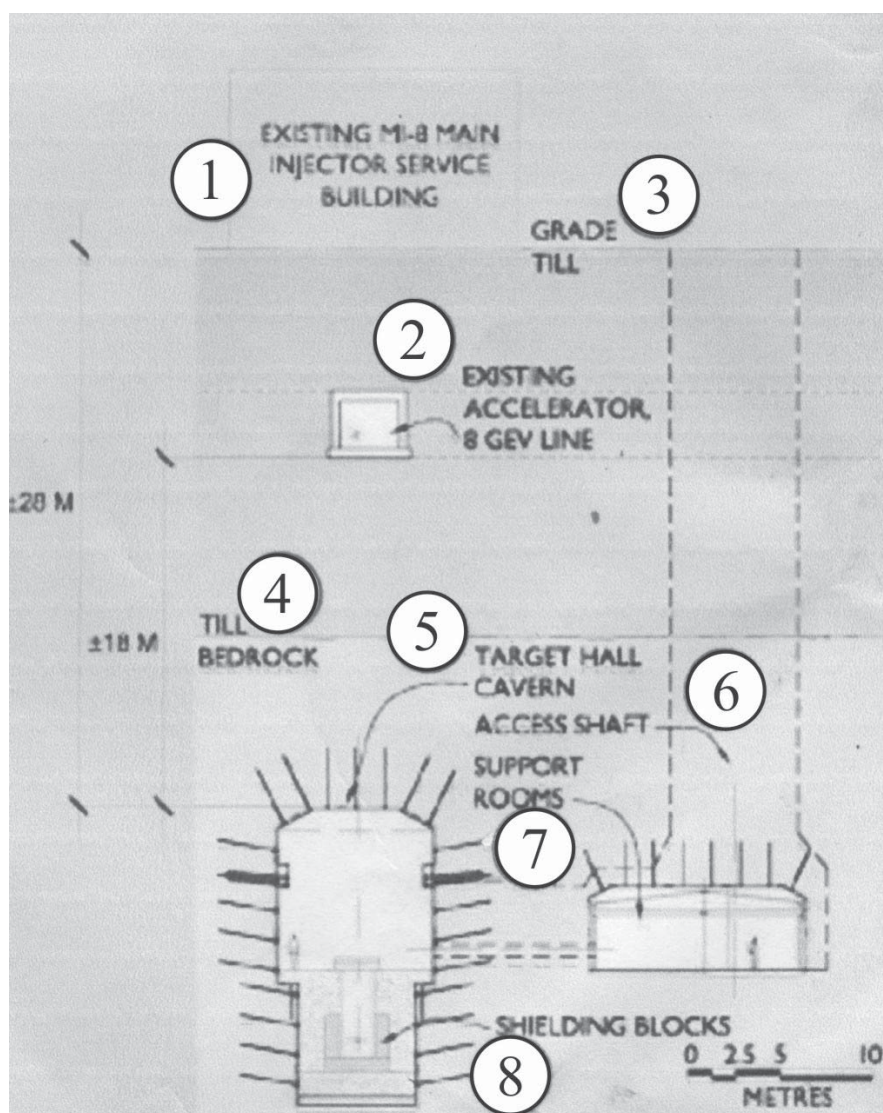
Рис. 4.16. Последовательность строительства подземной полости зала мишени «Target Hall» лаборатории Фермилаб 1 – существующее здание служб главного инжектора; 2 – существующий ускоритель; 3 – уровень валунной глины; 4 – уровень скальных пород; 5 – полость зала мишени; 6 – вертикальная шахта; 7 – вспомогательные камеры; 8 – блоки защиты оборудования
