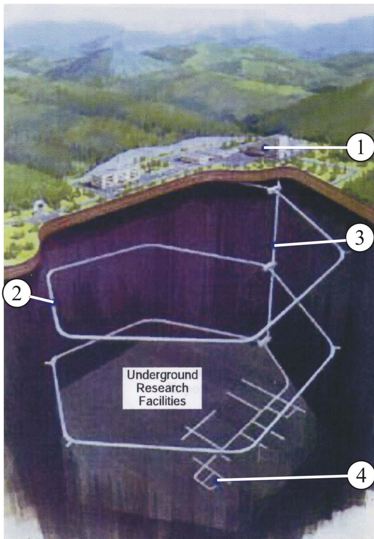
Рис. 3.41. Подземный комплекс лаборатории Хоронобе (Япония)
