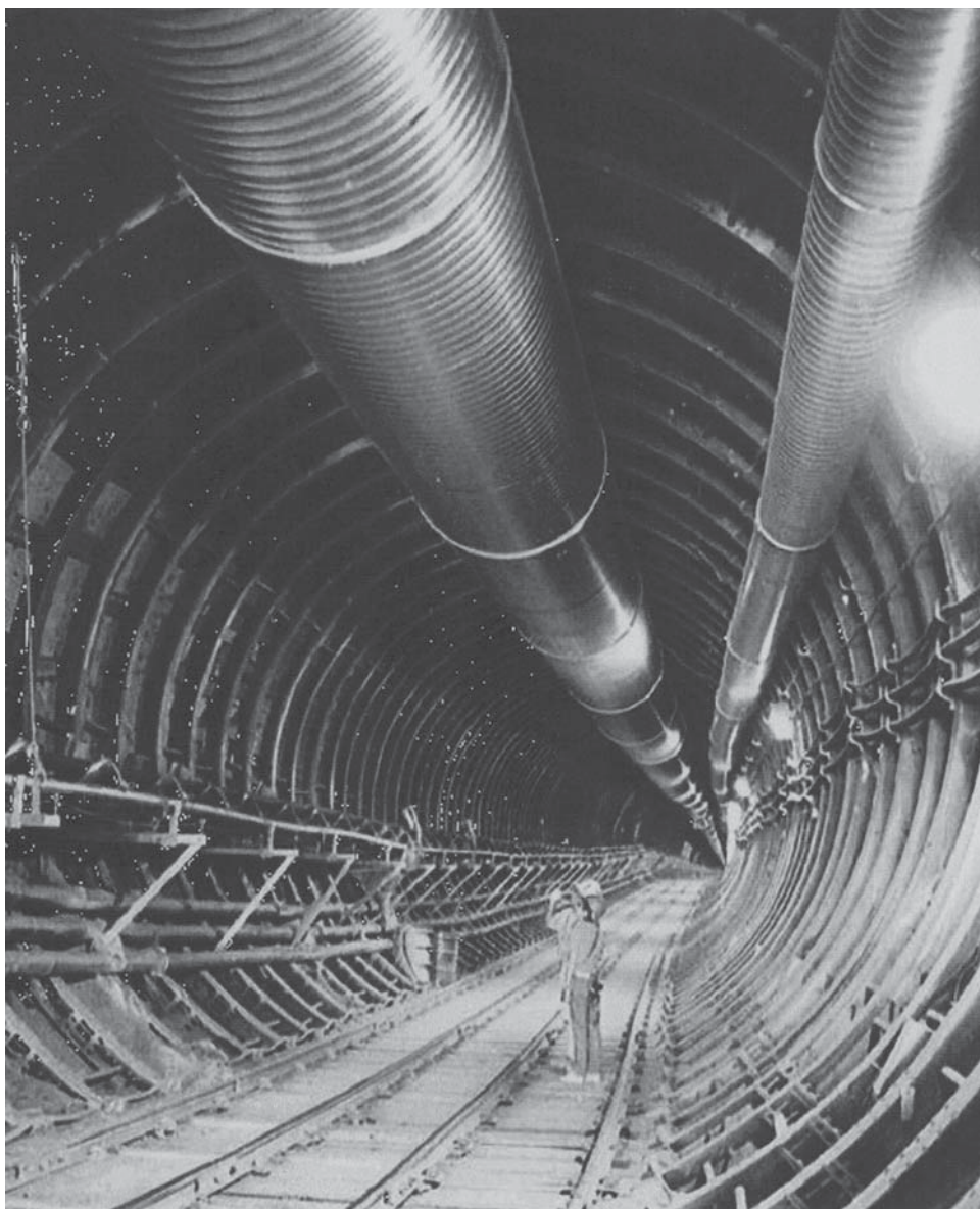
Рис. 3.13. Разведочный туннель после установки металлической крепи
