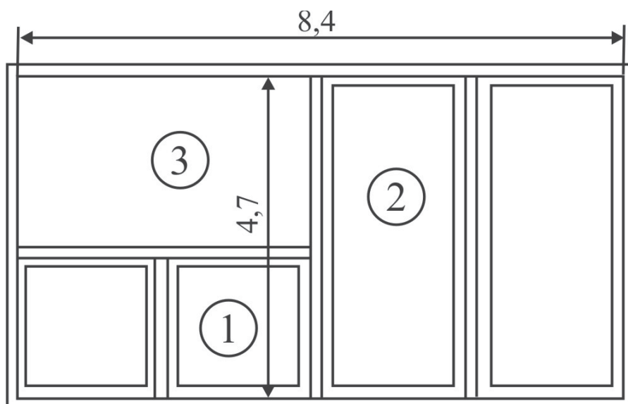
Рис. 4.21. Сечение ствола Ятес после реконструкции
