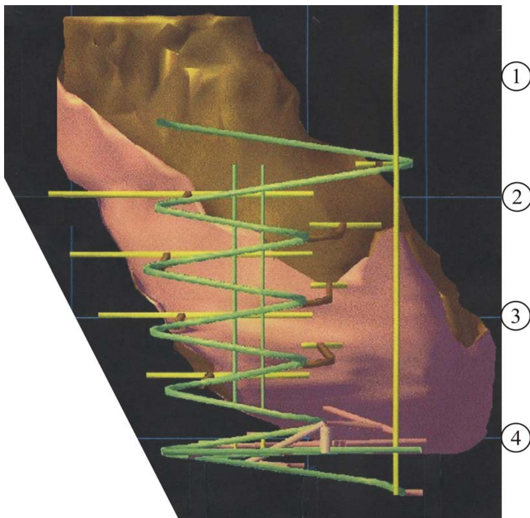
Рис. 4.51. Вскрытие нижней части месторождения шахты Пихасалми
