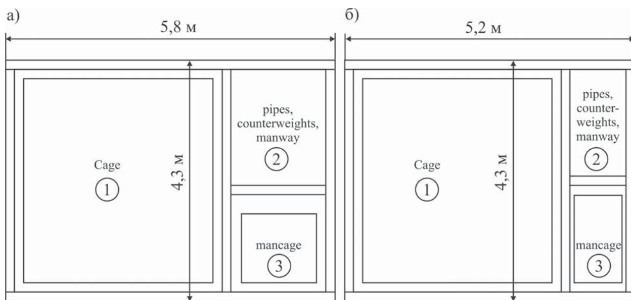
Рис. 4.22. Сечения стволов Росс и №6 после реконструкции
