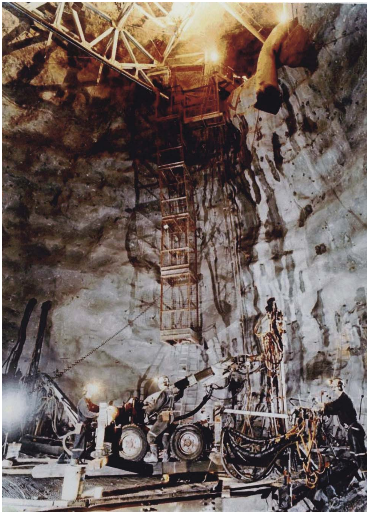
Рис .4.78. Проходка камеры детектора
