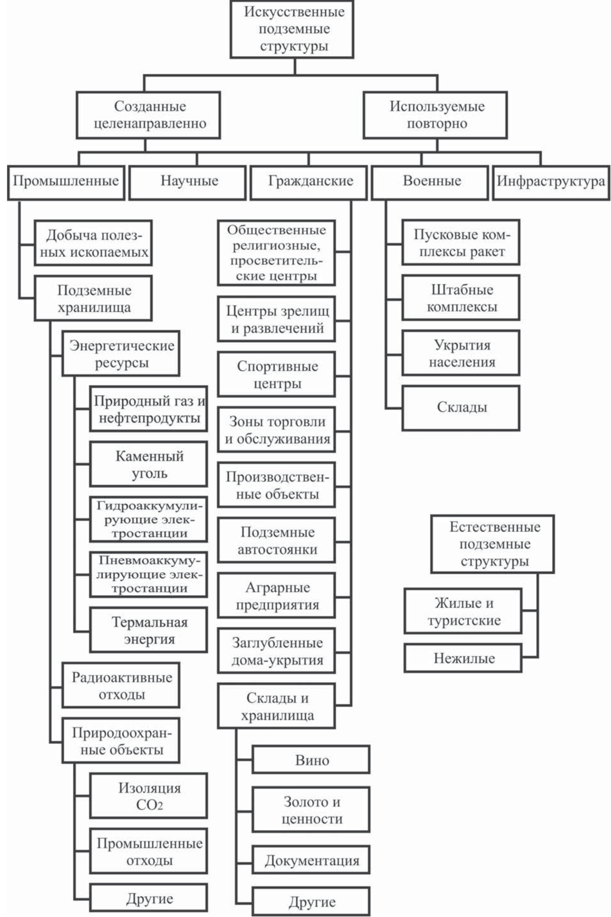
Рис. 1.1. Классификация подземных структур по назначению
