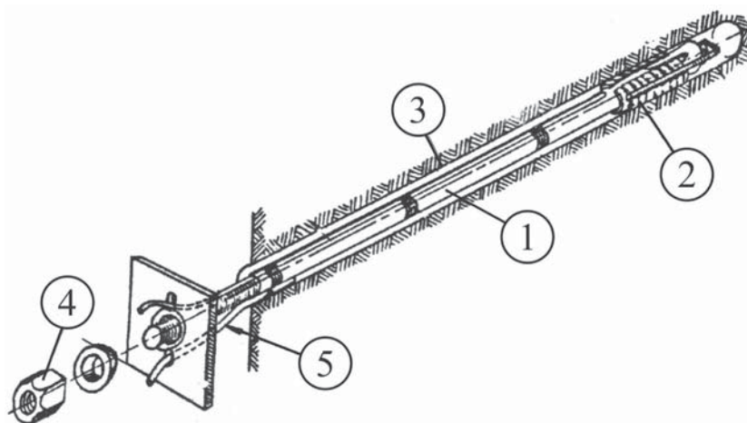
Рис. 1.19. Конструкция типичного анкерного болта
