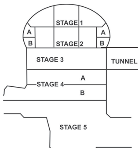
Рис. 1.12. Стадии строительства подземной гидроэлектростанции в Рио-Гранде (Аргентина)
