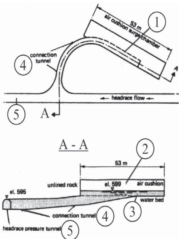
Рис. 2.53. План и разрез амортизирующей камеры 1 – амортизирующая камера; 2 – воздушная подушка; 3 – слой воды; 4 – соединительный туннель; 5 – головной напорный туннель станции
