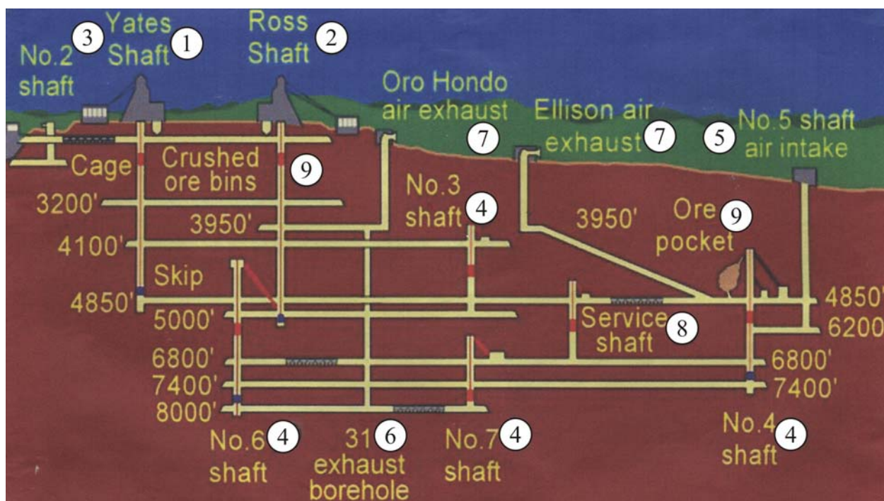
Рис. 4.19. Схема вскрытия месторождения шахты Хоумстейк
