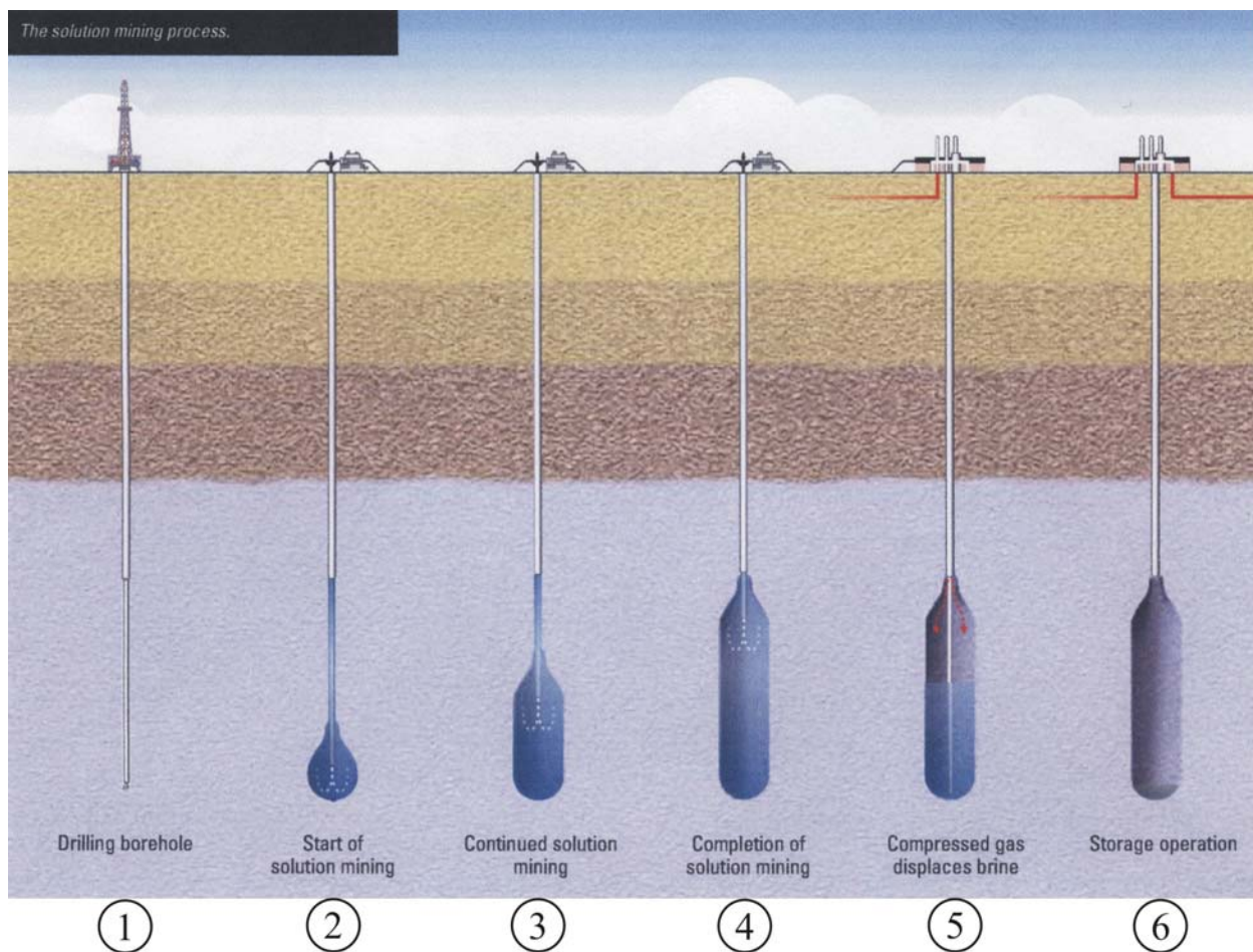
Рис .2.57. Порядок подготовки полости в соляном слое
