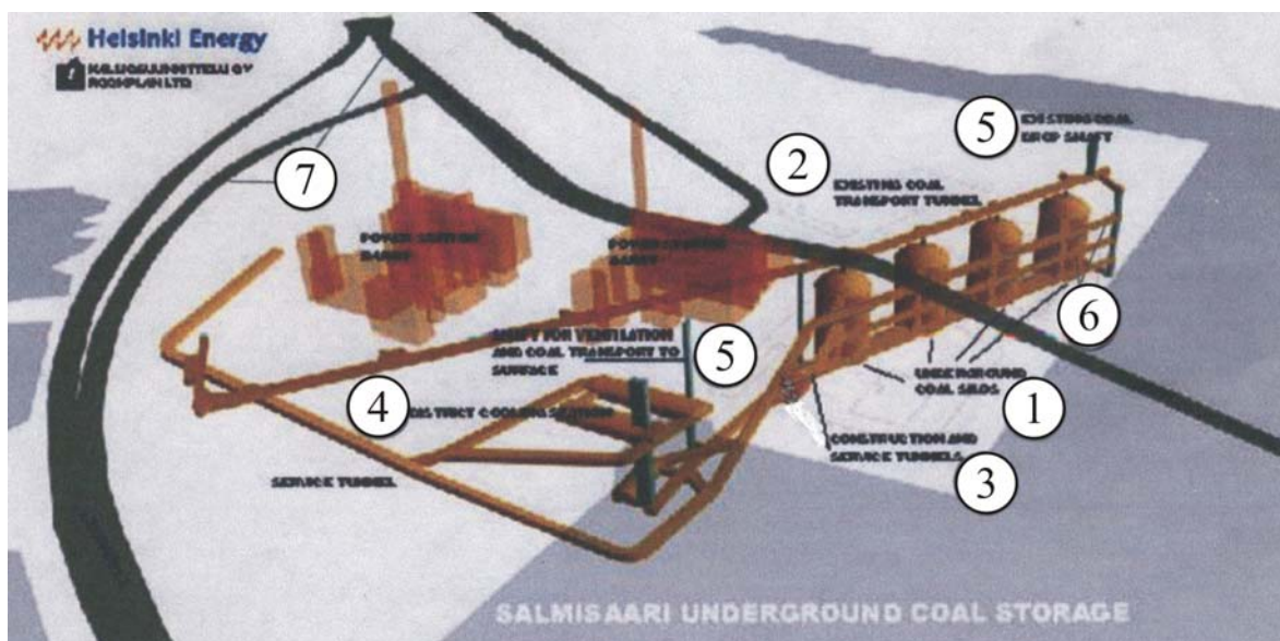
Рис. 2.28. Схема расположения подземных угольных бункеров
