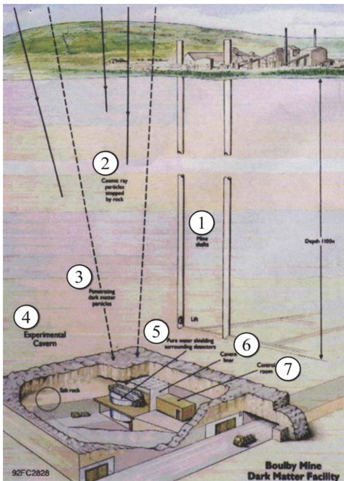
Рис. 4.57. Схема вскрывающих горных выработок шахты Балби и подземной физической лаборатории
