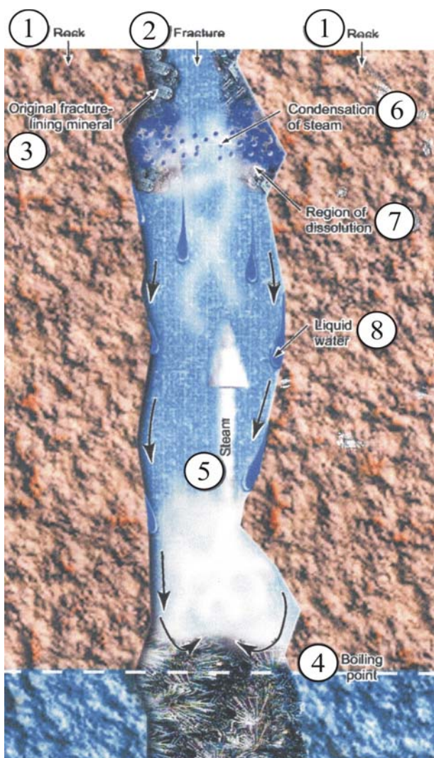
Рис. 3.48. Зона пород, примыкающих к туннелю хранения, нарушенных горными работами
