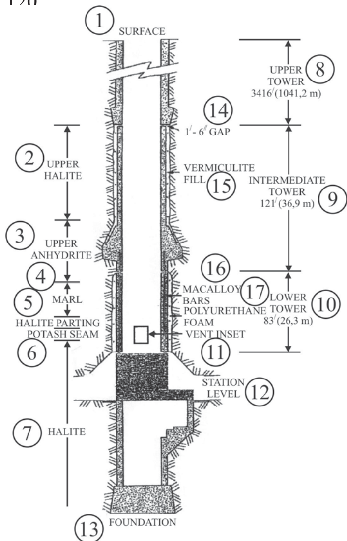
Рис. 4.62. Крепь ствола, установленная при его проходке
