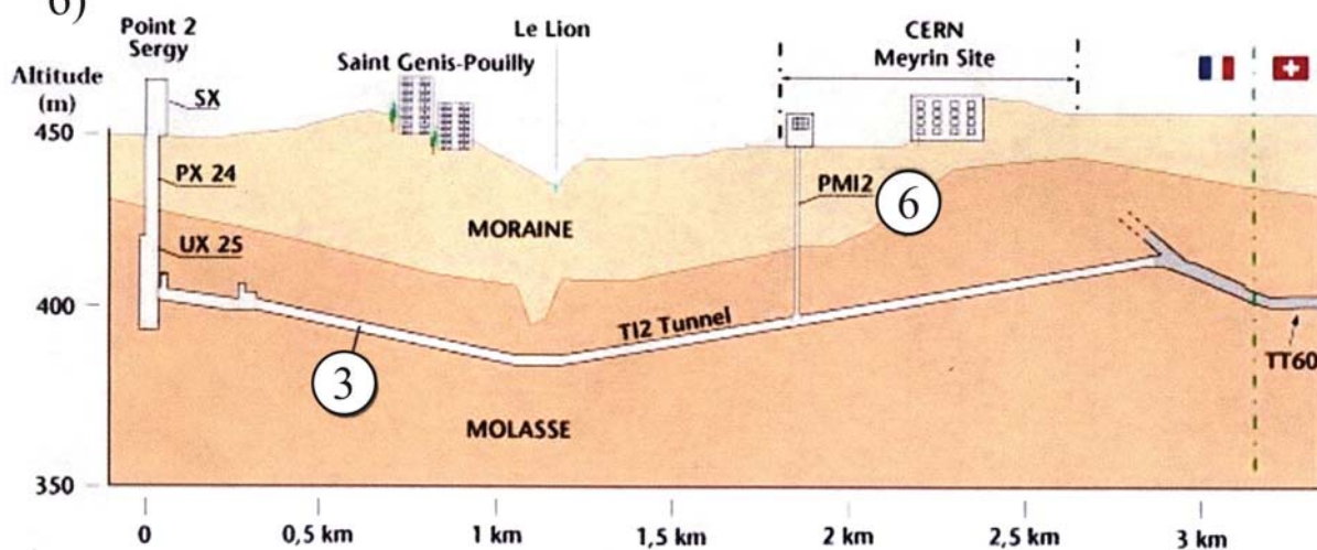
Рис. 4.97. Схемы туннелей T12 и T18 при реконструкции комплекса ускорителя LEP/LHC
