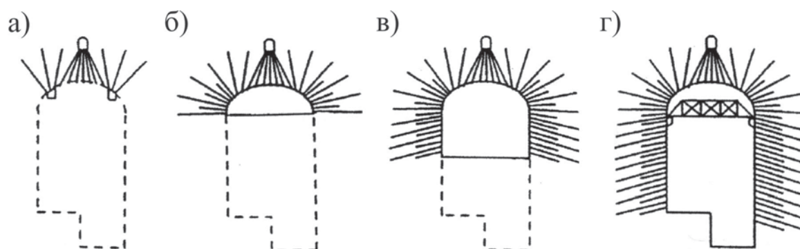
Рис. 1.21. Стадии проходки и установки анкерной крепи в полости большого сечения
