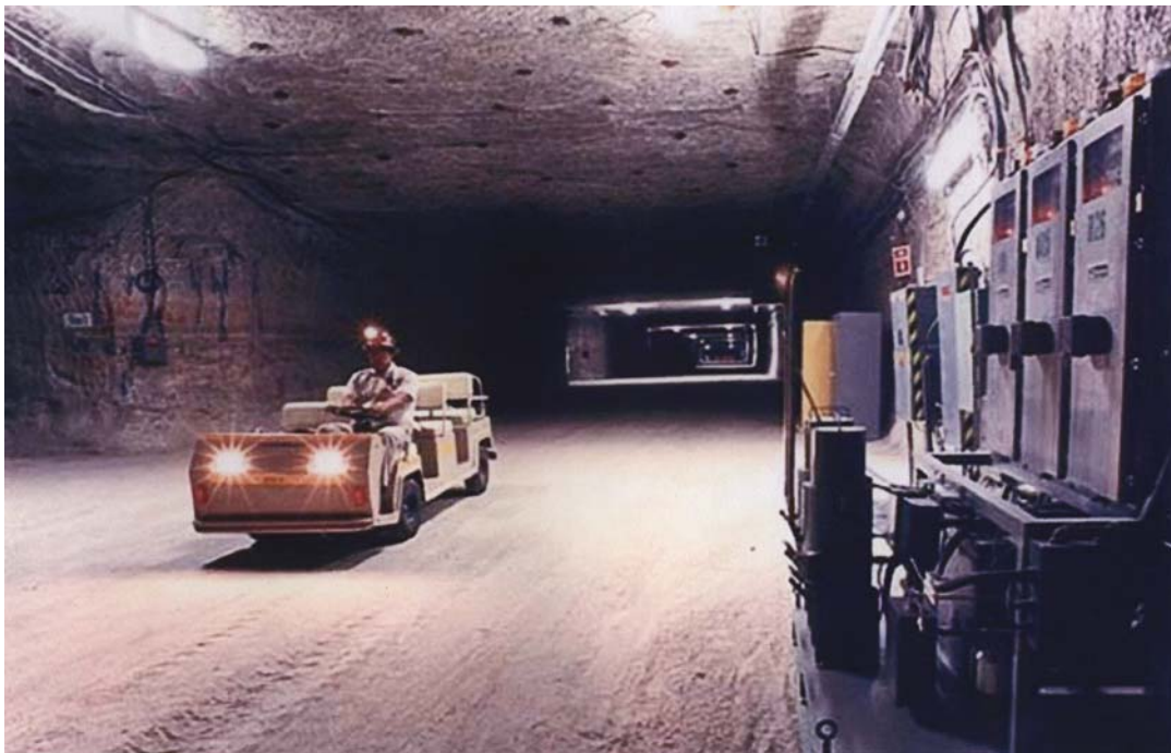
Рис. 3.26. Туннель панелей хранения отходов
