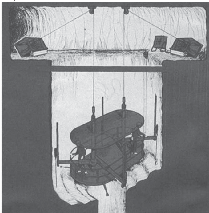
Рис. 1.11. Расположение оборудования при расширении шахты а – круглое сечение; б – эллиптическое сечение
