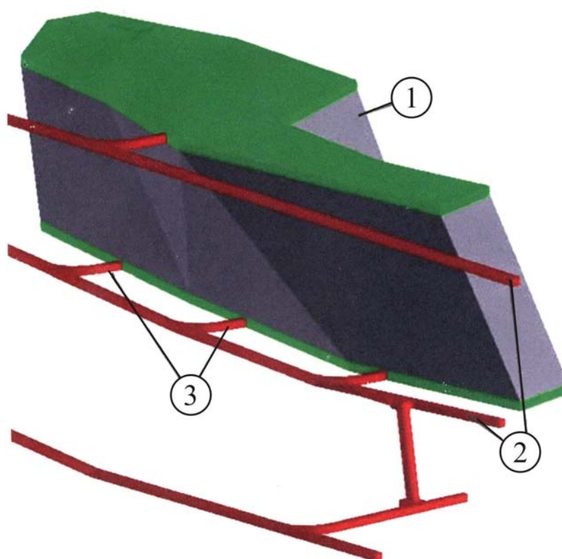
Рис. 4.20. Схема вскрытия рудного тела участковыми выработками
