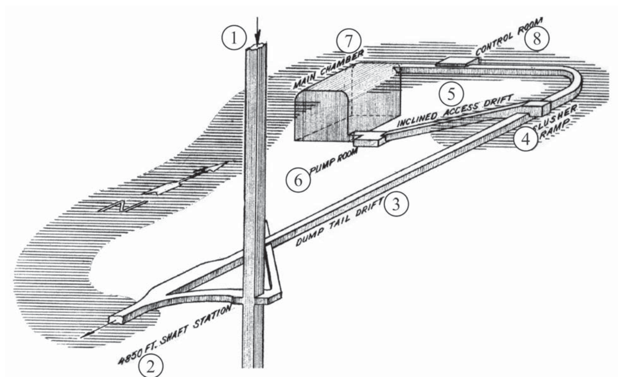
Рис. 4.23. Схема подземной нейтринной лаборатории на горизонте 4850 футов
