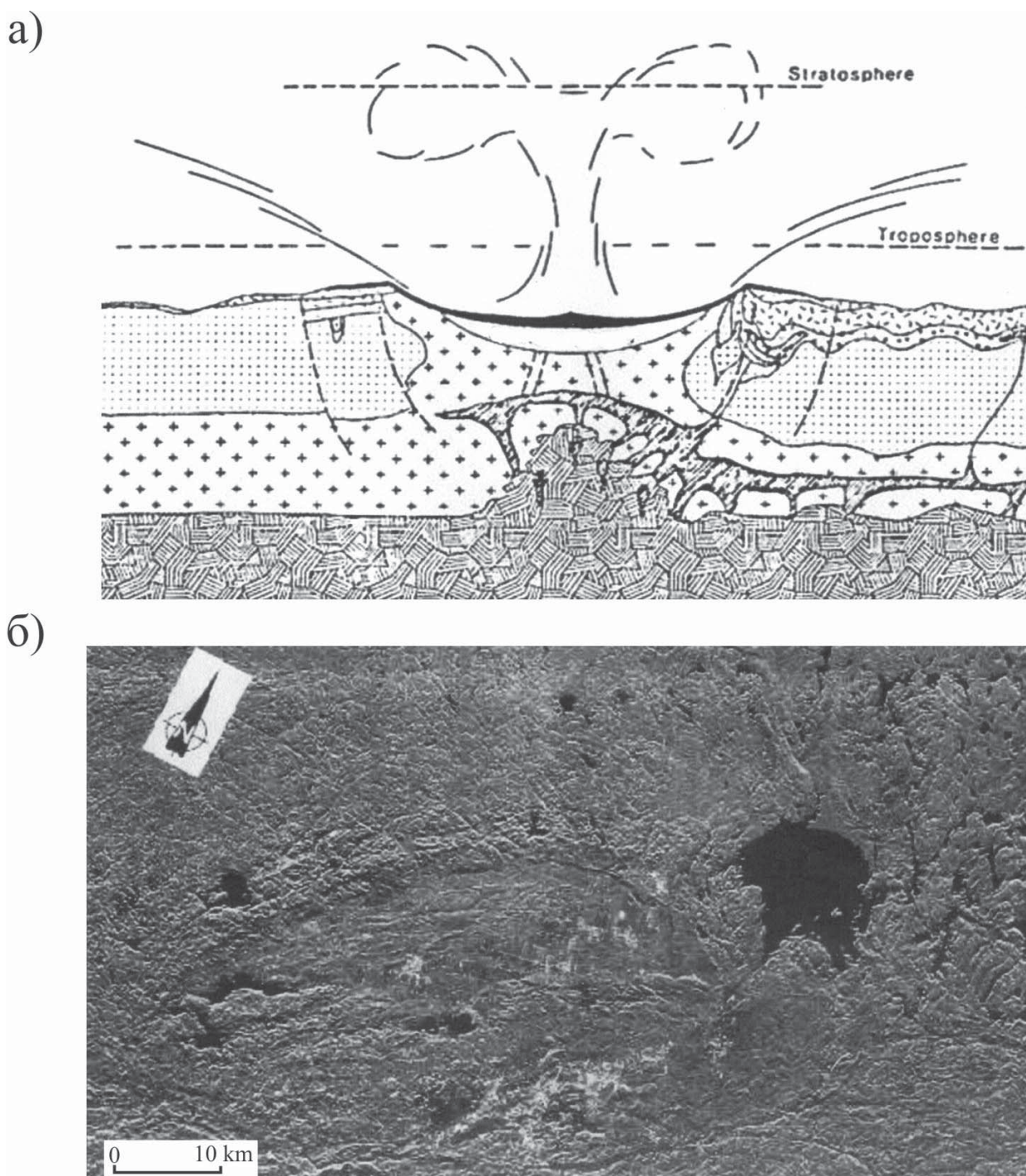
Рис. 4.68. Схема образования месторождения Садбери а – образование кратера при ударе метеорита; б – вид со спутника на контуры кратера (справа – озеро Ванапитаи (Wanapitai)), в – план контуров кратера; 1 – город Садбэри; 2 – медно-никелевые шахты; 3 – озеро Ванапитаи
