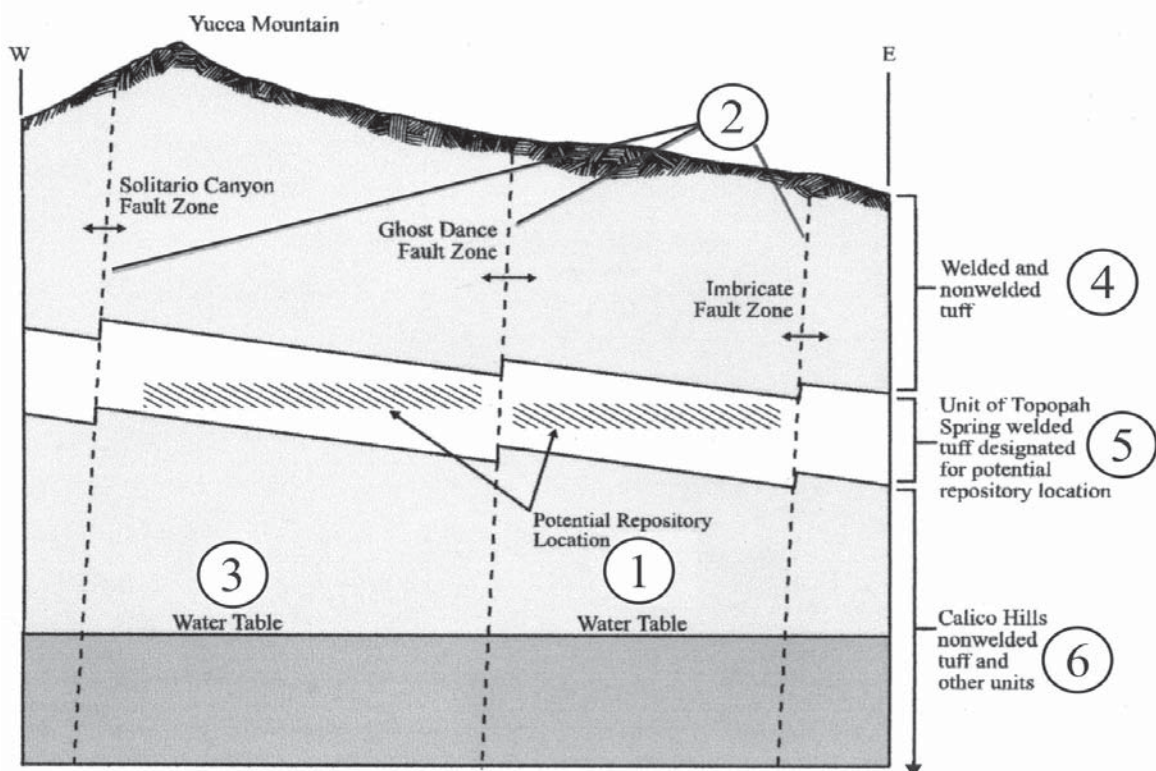
Рис. 3.15. Схема основных геологических нарушений и блоков в районе строительства хранилища Юкка Маунтейн
