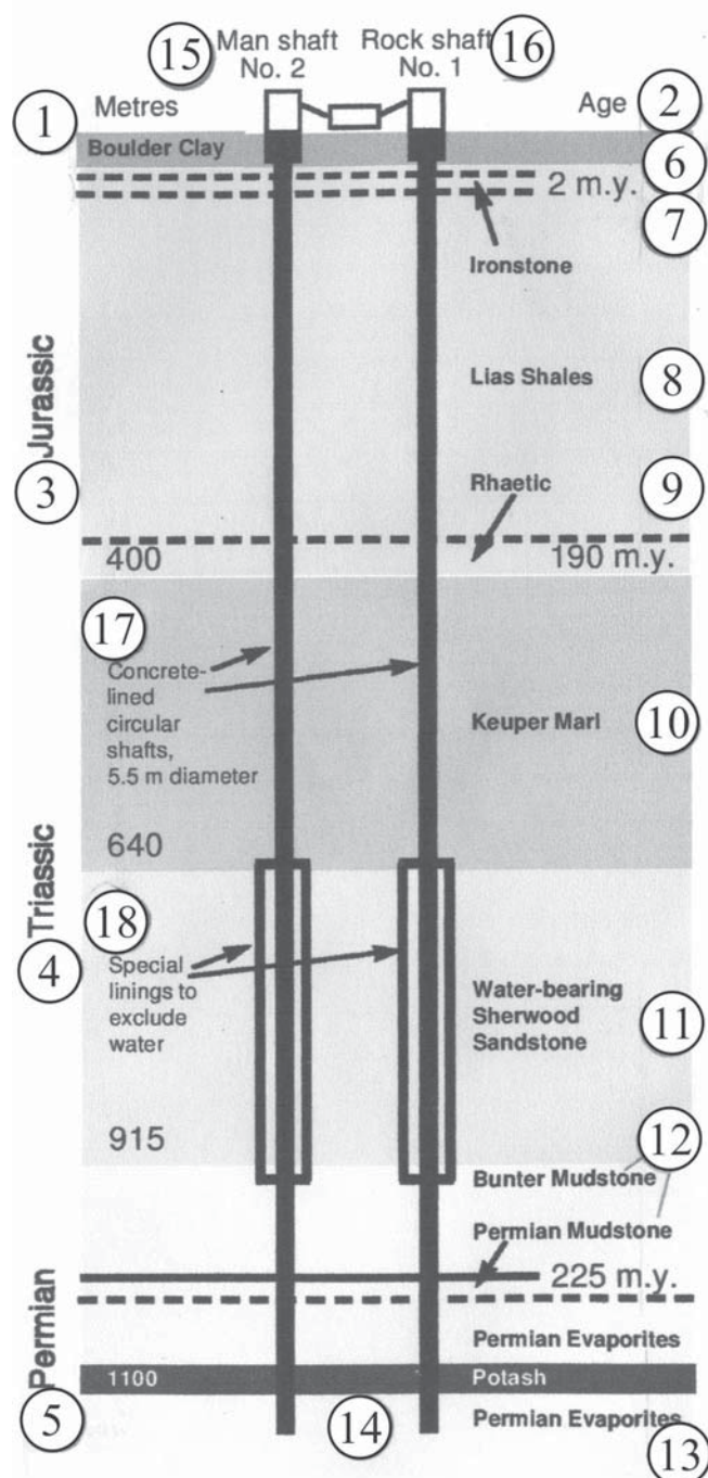
Рис. 4.61. Геологический разрез по шахтным стволам
