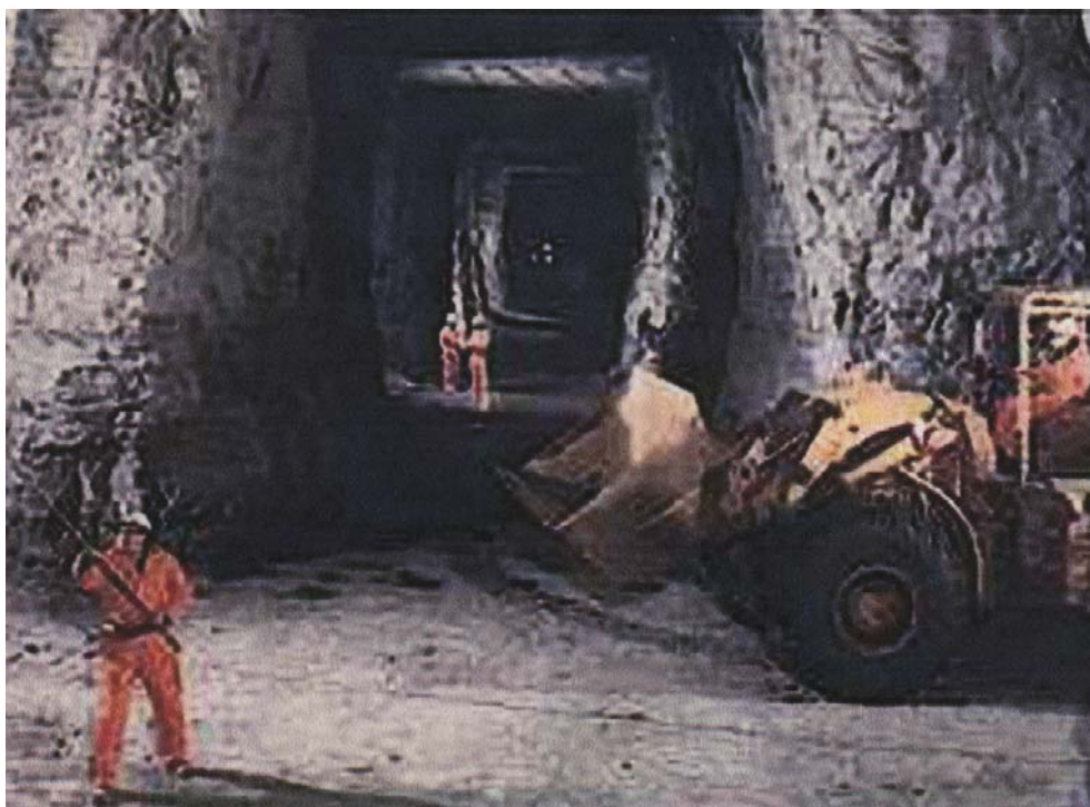
Рис. 2.10. Строительство полости
