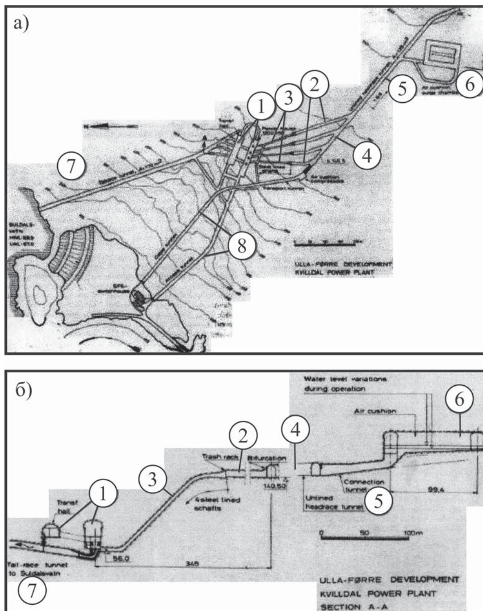
Рис. 2.44. Подземный комплекс гидроэлектростанции Квиллдал а – план; б – разрез по основным туннелям и полостям; 1 – машинные залы; 2 – горизонтальные туннели; 3 – наклонные шахты подачи воды; 4 – распределительный туннель; 5 – головной туннель; 6 – амортизирующая камера; 7 - хвостовой туннель; 8 – подводящие туннели
