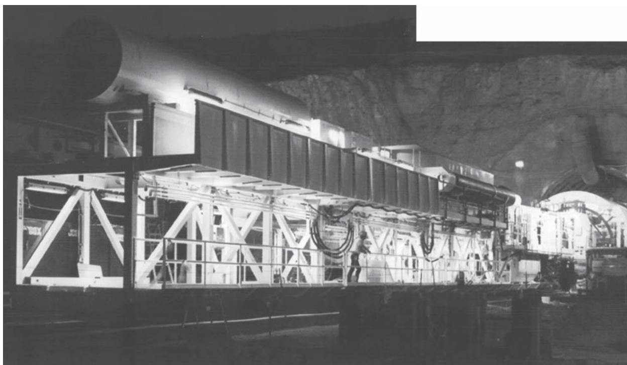
Рис. 3.10. Начало проходки разведочного туннеля буровой туннельной машиной
