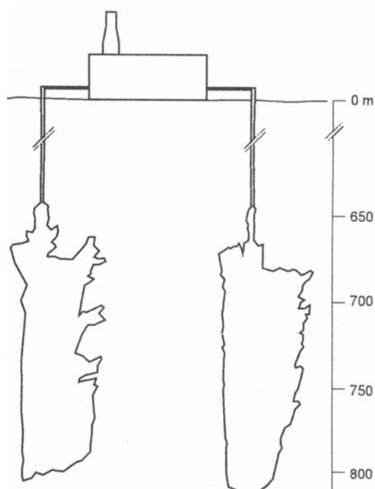
Рис. 2.59. Соляные полости станции Хантдорф (полости и здание станции выполнены в одном масштабе)
