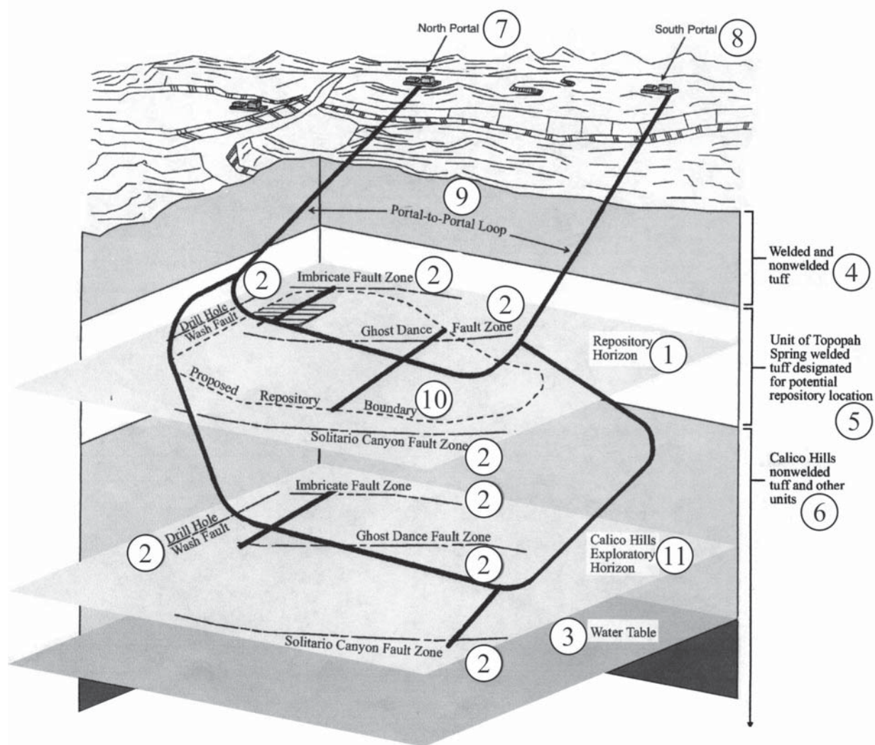
Рис. 3.16. Схема расположения основных туннелей и хранилища Юкка Маунтейн
