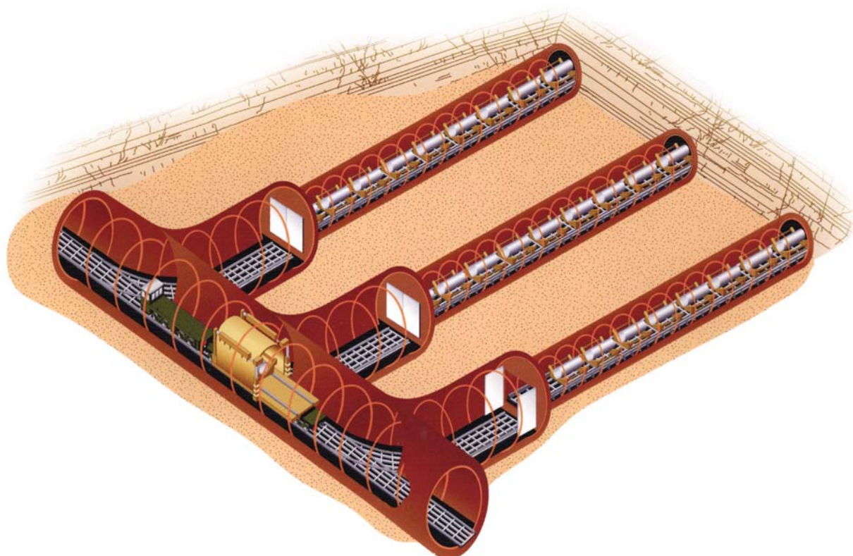
Рис. 3.17. Конструкция транспортных туннелей и туннелей хранения
