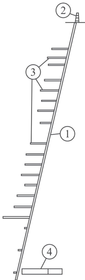
Рис. 4.3. Схема вскрытия шахты Саудан 1 – ствол; 2 – поверхностный комплекс; 3 – вскрывающие выработки горизонтов; 4 - лабо- ратория Саудан-2
