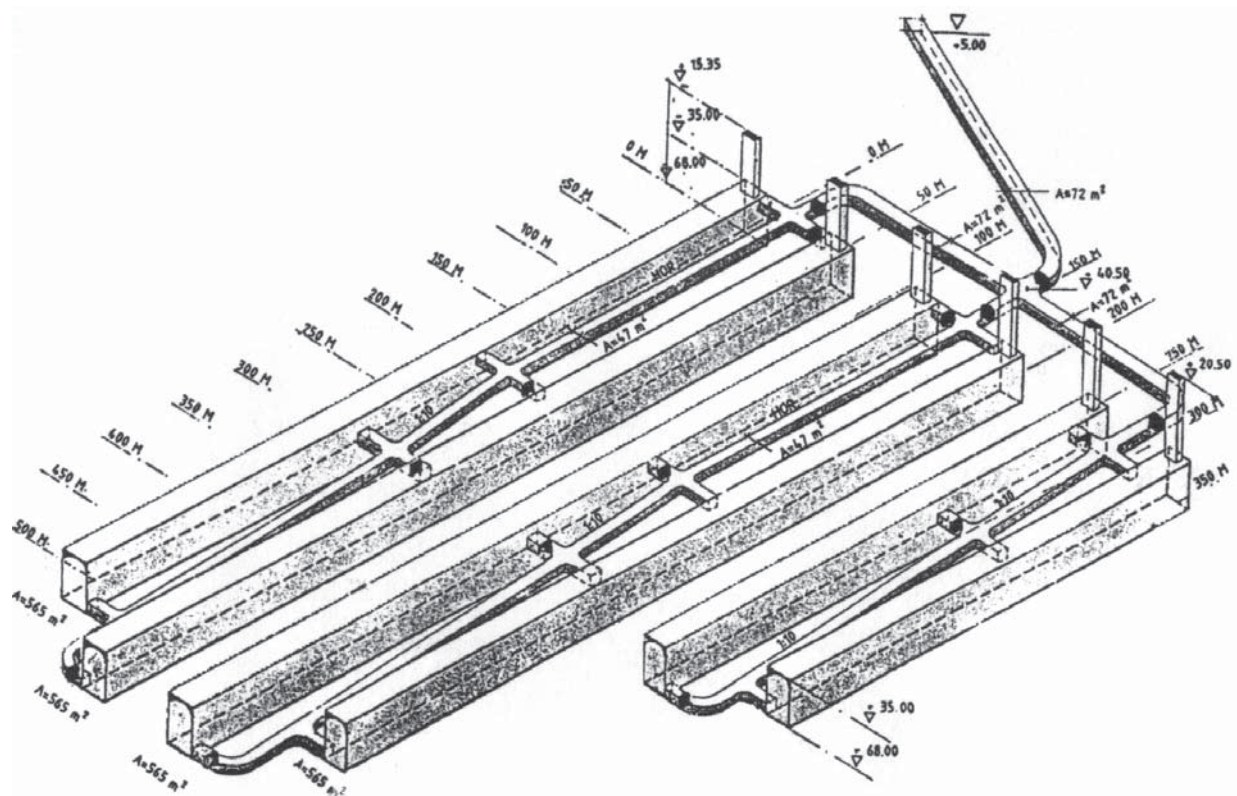
Рис. 2.12. Хранилище нефти в Монгстаде
