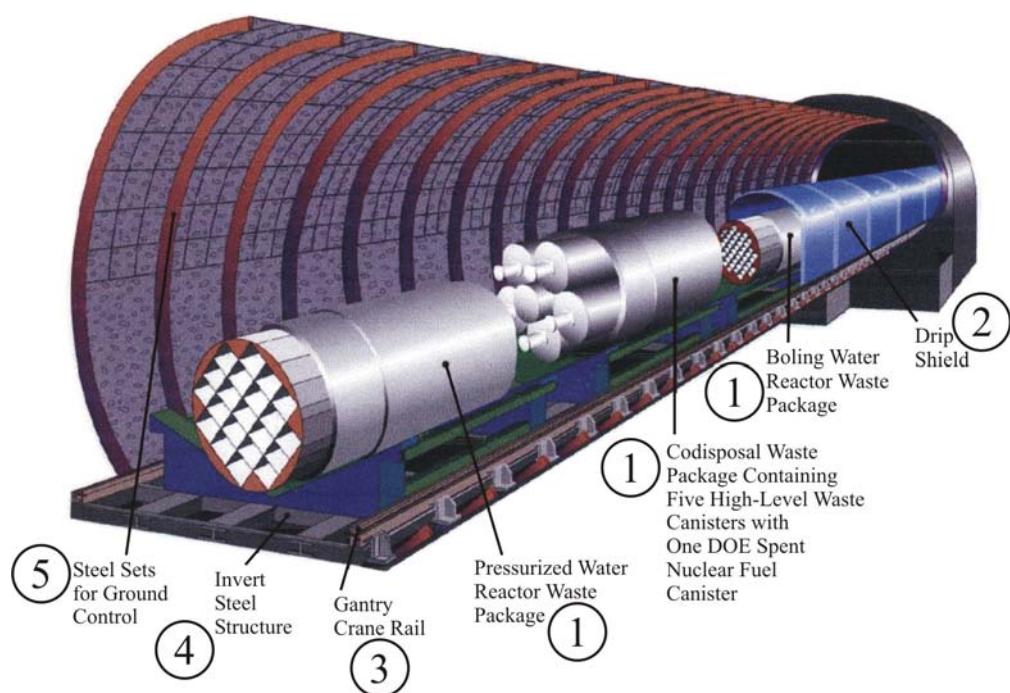
Рис. 3.20. Расположение контейнеров с отходами в туннеле хранения
