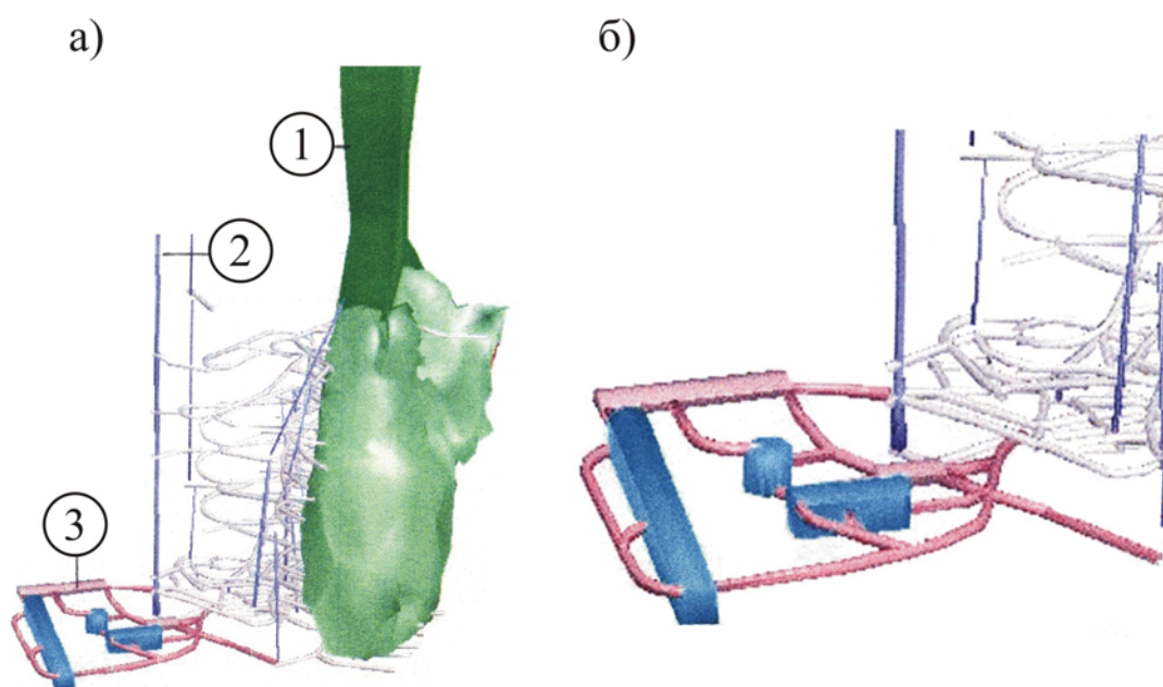
Рис. 4.52. Перспективный комплекс научных лабораторий на гор. 1440 м
