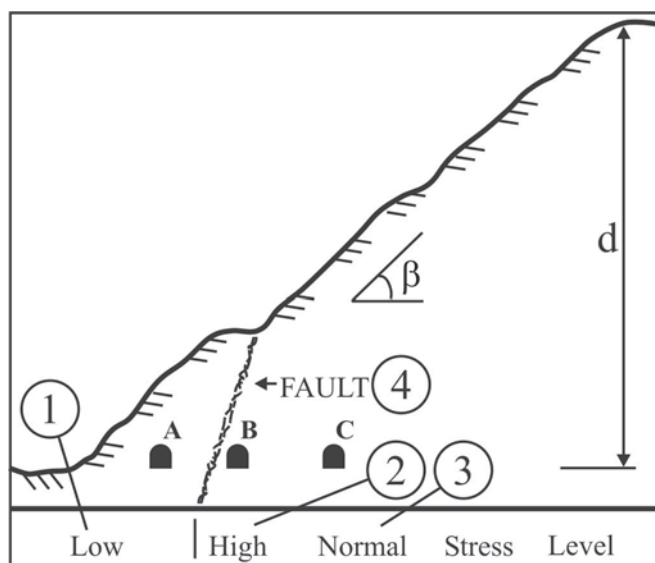
Рис. 1.4. Зависимость уровня напряженного состояния горных пород от места расположения подземной полости
