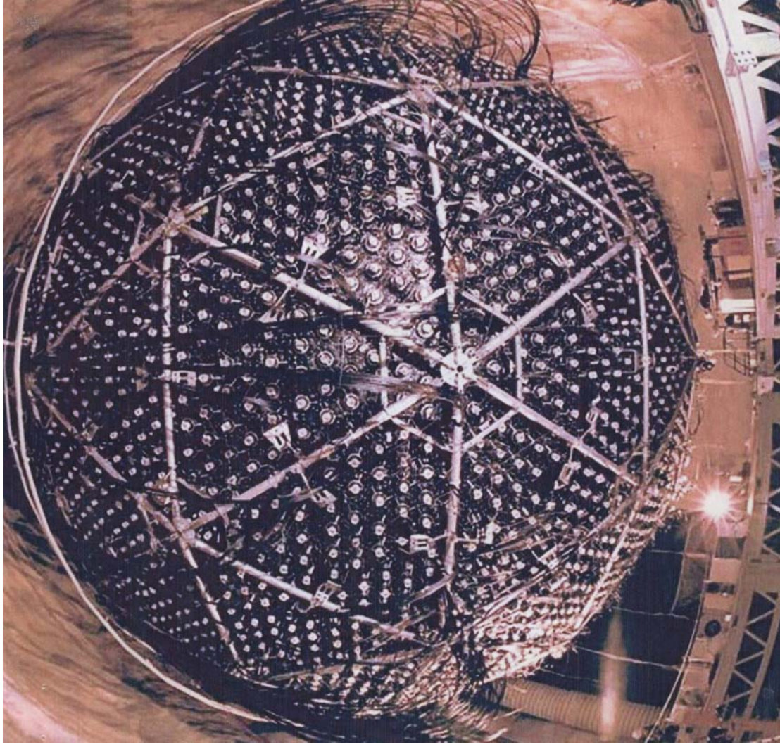
Рис. 4.74. Наружный вид детектора SNO
