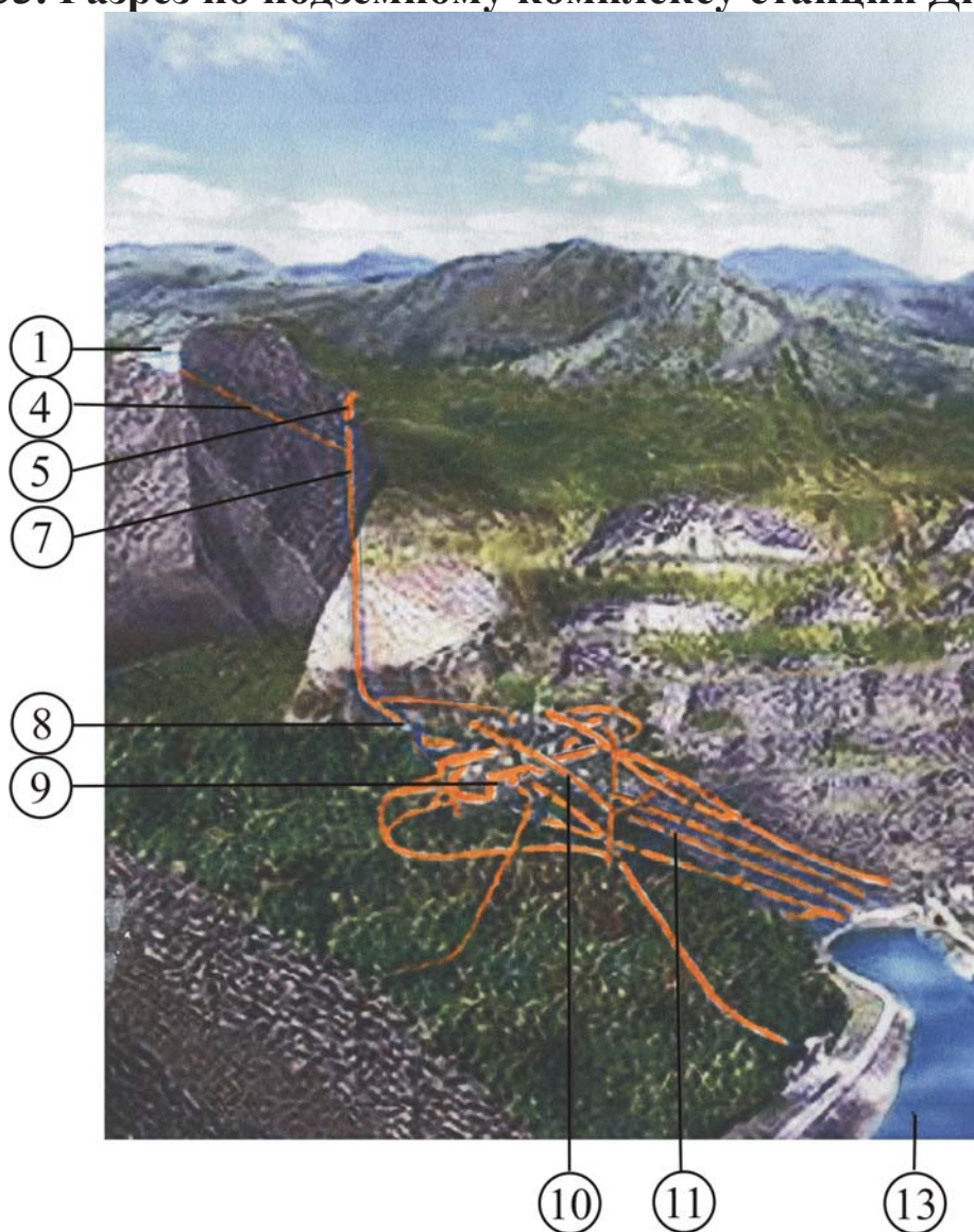
Рис. 2.34. Расположение основных объектов станции Динорвиг в окружающем ландшафте
