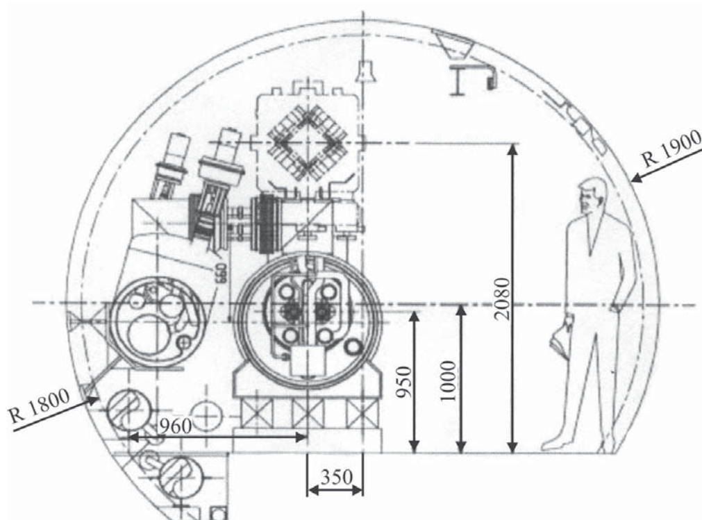
Рис. 4.93. Схема сечения туннеля ускорителя
