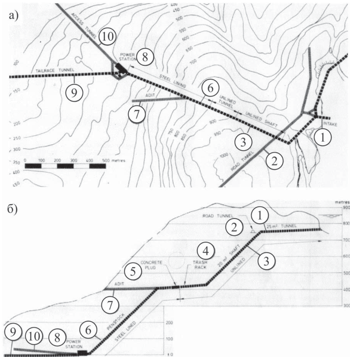
Рис. 2.43. Расположение комплекса туннелей гидроэлектростанции Мауранджер
