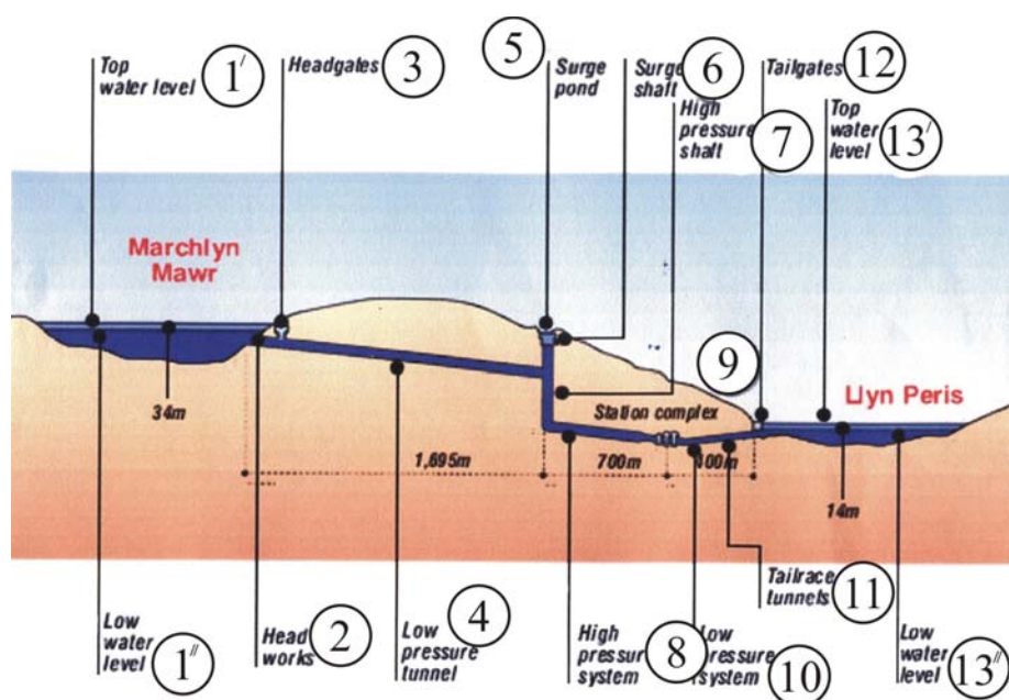
Рис. 2.33. Разрез по подземному комплексу станции Динорвиг
