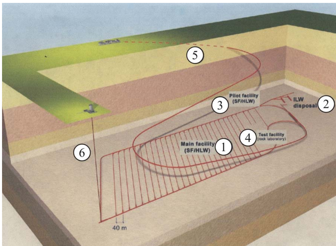
Рис. 3.38. Схема подземного комплекса хранилища ядерных отходов (Швейцария)
