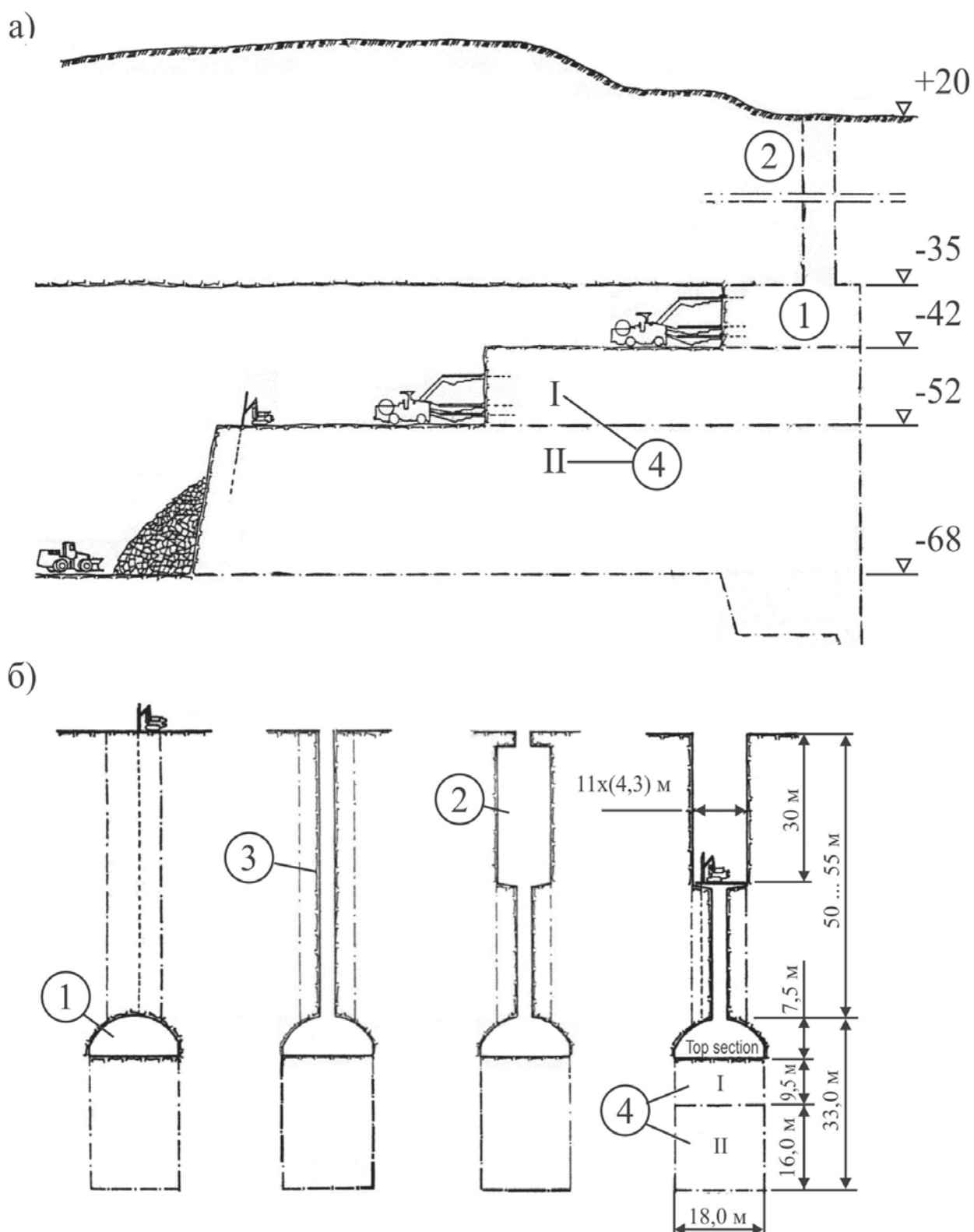
Рис. 1.10. Стадии проходческих работ по строительству полости большого размера
