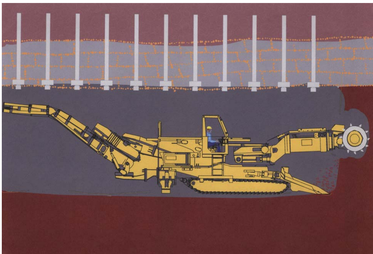
Рис. 1.24. Схема работы проходческого комбайна
