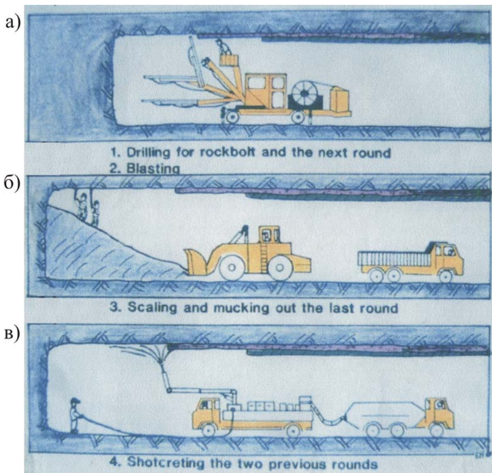
Рис. 1.13. Последовательность операций при проходке подземной полости буровзрывным способом
