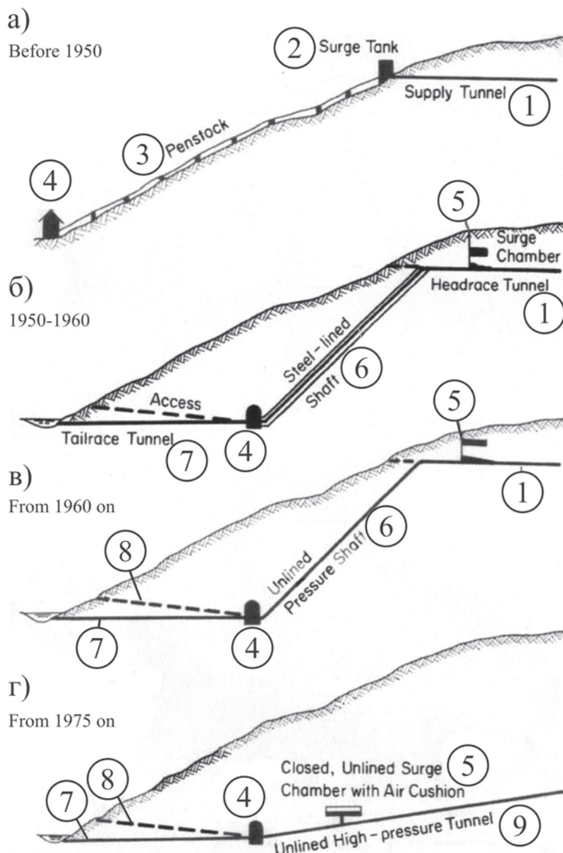
Рис. 2.41. Этапы совершенствования структур подземных гидроэлектростанций
