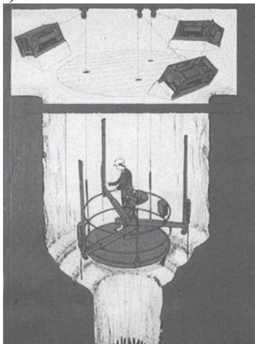
Рис. 1.11. Расположение оборудования при расширении шахты а – круглое сечение; б – эллиптическое сечение
