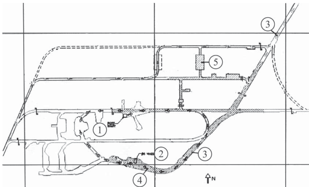
Рис. 4.26. Вариант размещения лабораторного комплекса на горизонте 4850 ф
