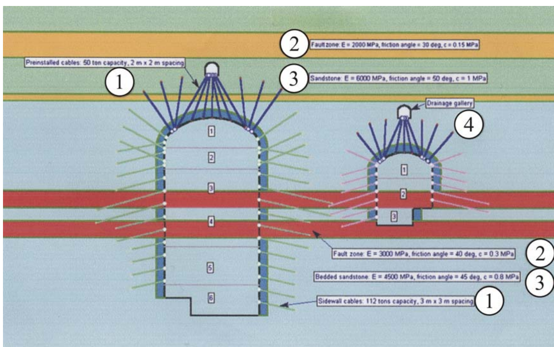
Рис. 1.8. Цифровая модель, показывающая схему необходимого усиления анкерной крепью пород, окружающих полости
