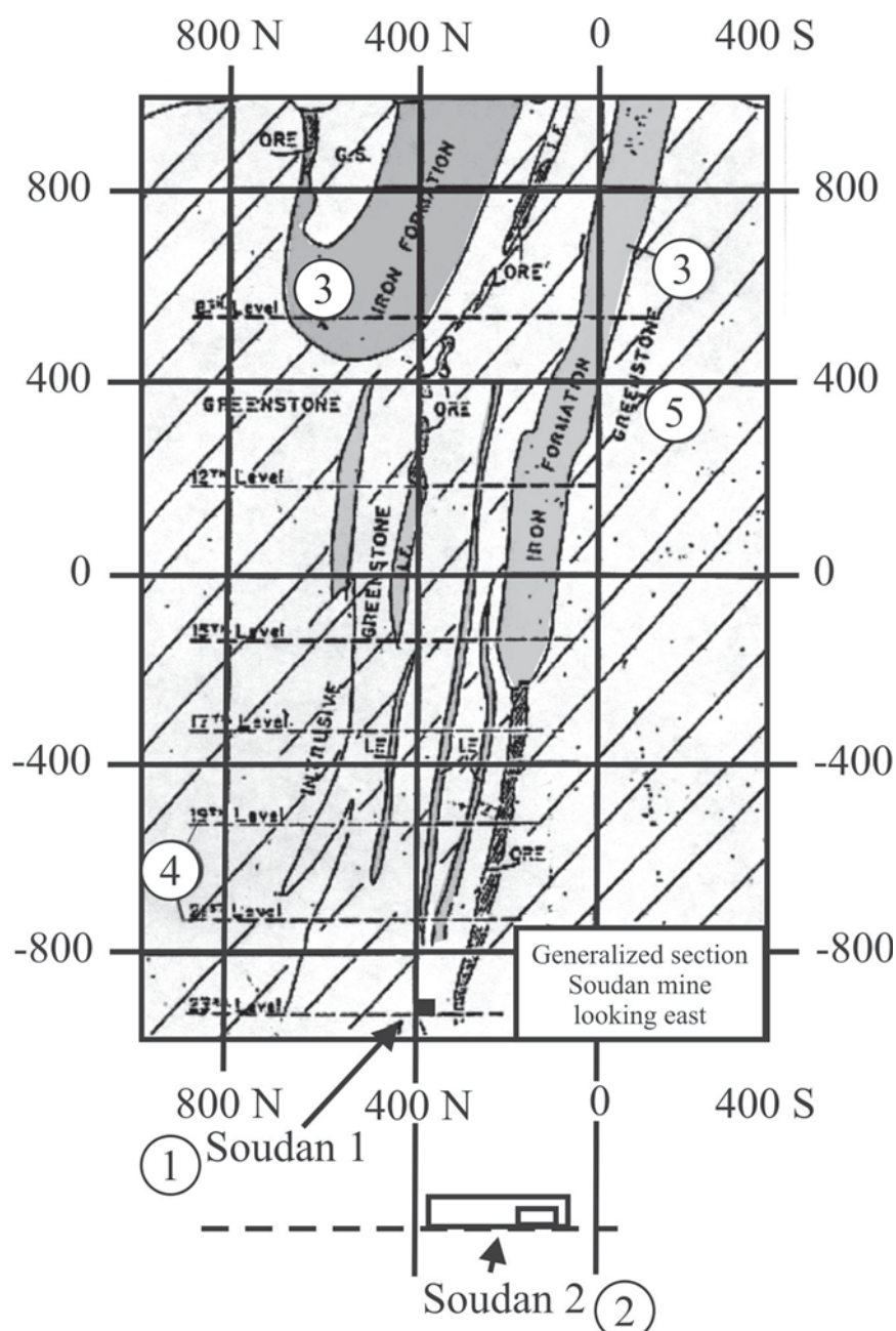
Рис. 4.1. Геологический разрез месторождения Саудан
