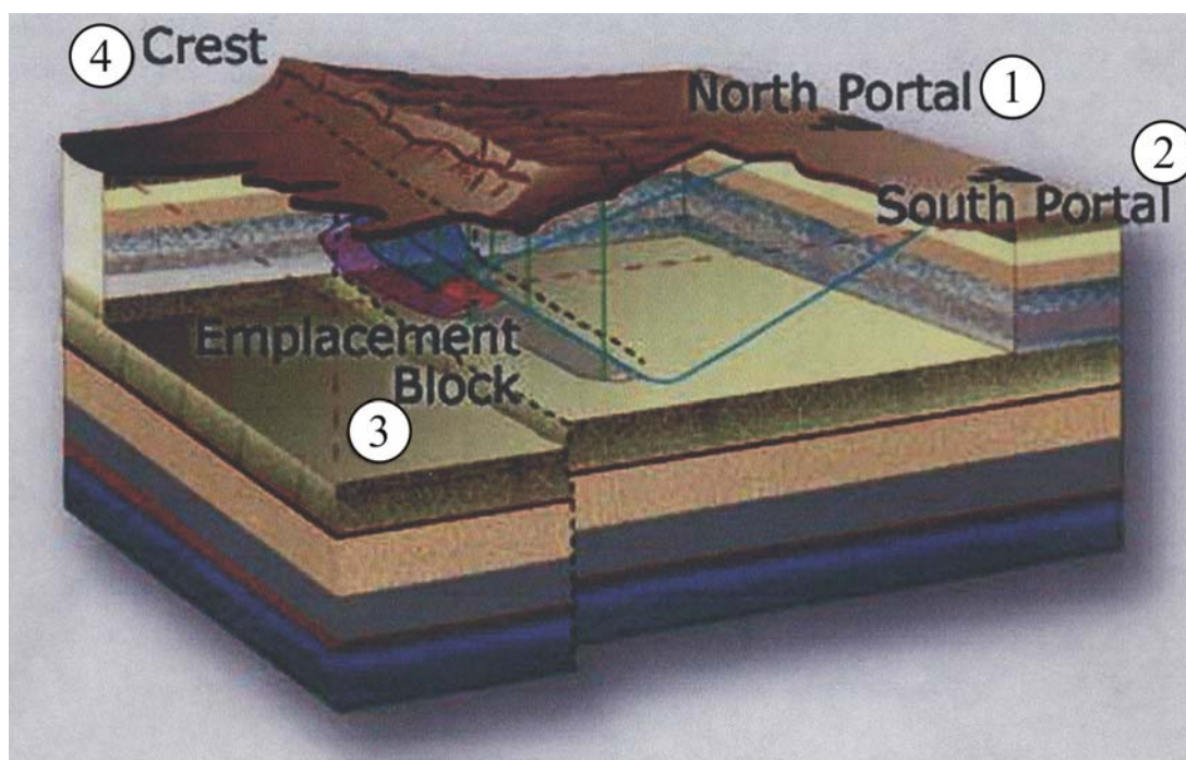
Рис. 3.7. Совмещенная схема геологических формаций и главного туннеля
