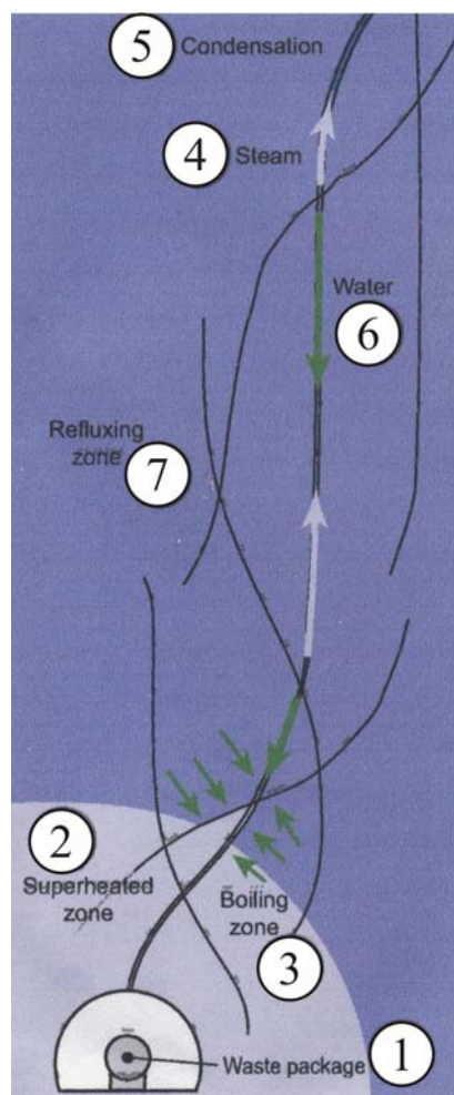
Рис. 3.49. Общая схема движения пароводяного потока в породах, перекрывающих туннель хранения отходов
