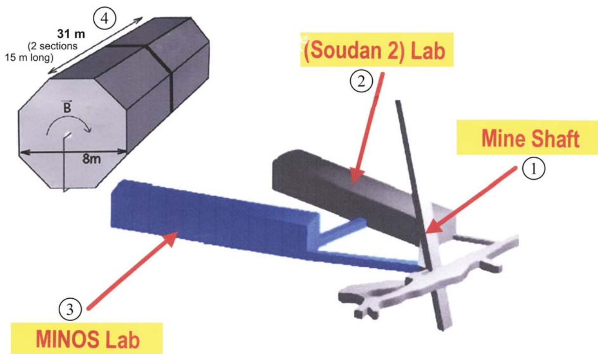
Рис. 4.11. Схема подземного лабораторного комплекса Саудан-2 (27 горизонт шахты)
