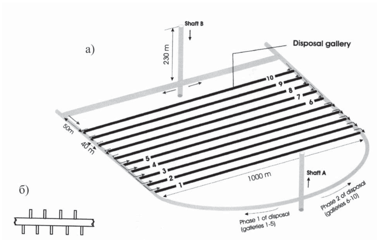
Рис. 3.37. Схема хранилища отходов в Бельгии
