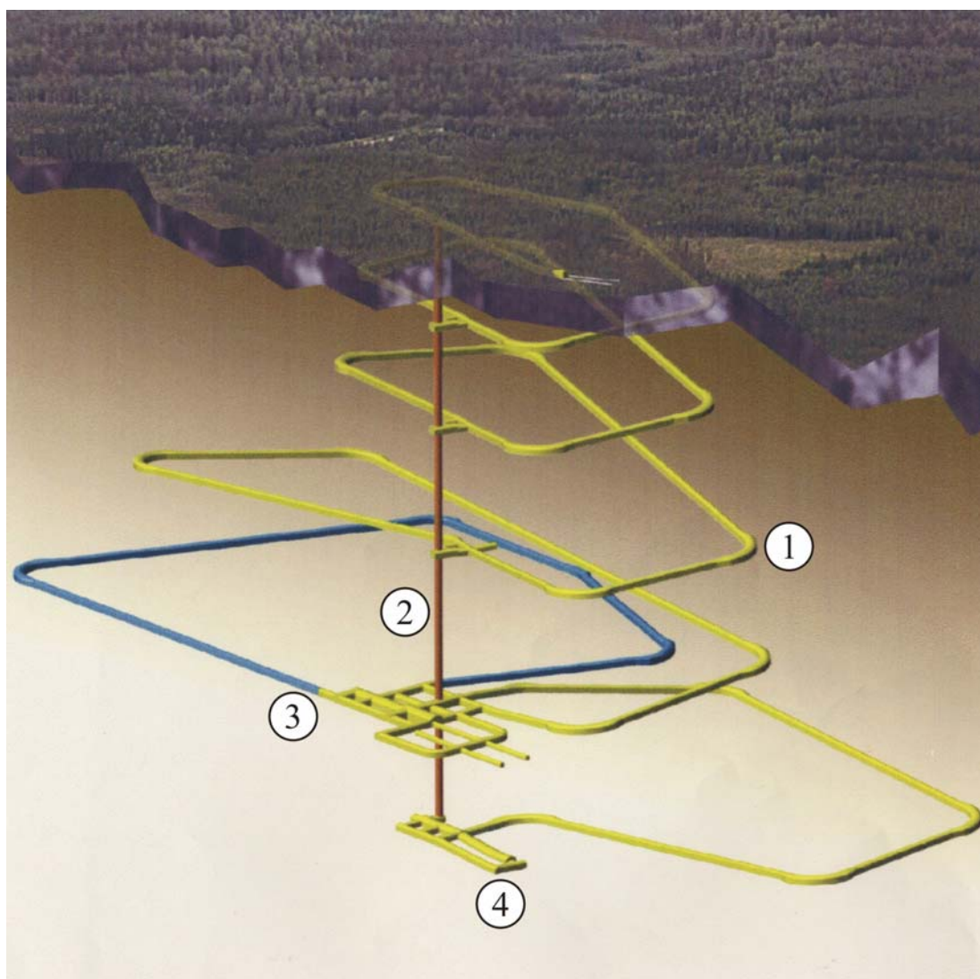
Рис. 3.43. Подземный комплекс лаборатории ONKALO (Финляндия)
