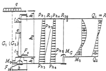
Черт. 3. Расчетная схема стены подвала
