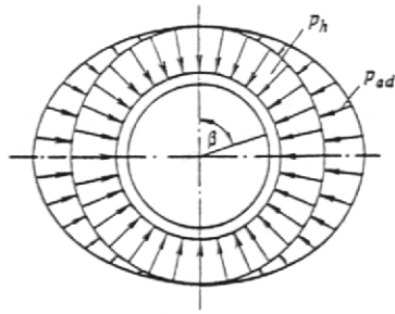
Черт. 5. Схема распределения основного p_h и дополнительного p_{ad} горизонтального давления грунта на круглый колодец
