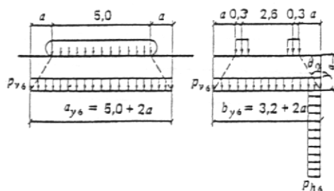
Черт. 6. Схема давления от гусеничной нагрузки НГ-60 при движении ее вдоль сооружения
