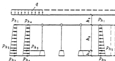
Черт. 2. Расчетная схема поперечной рамы подвала
