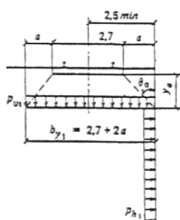
Черт. 3. Схема распределения давления от подвижного состава железных дорог
