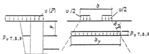
Черт. 7. Схема давления от нагрузок АК, НК-80 и НГ-60 при движении их поперек сооружения
