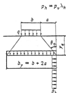
Черт. 2. Схема распределения давления от полосовой нагрузки
