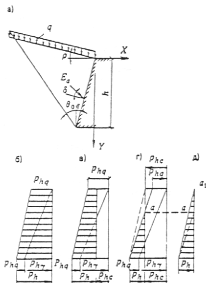
Черт. 1. Схема давления грунта
